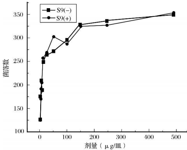
图 1 在不同浓度的多壁碳纳米管作用下 TA97 回变菌落数的散点图
