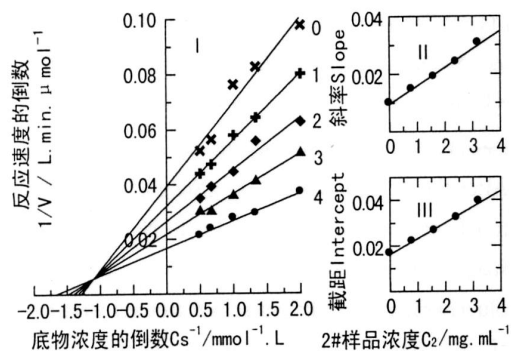
图3 2^{\#} 样品对蘑菇酪氨酸酶抑制类型和抑制常数的测定 Fig.3 Determination of the inhibitory type and inhibition constant of 2^{\#} sample on tyrosinase 曲线0~4 分别代表测活体系中加入的 2^{\#} 样品的浓度分别为 0、0.8、1.6、2.4 和 3.2 mg/mL。
