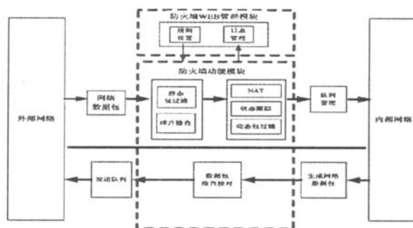
图 2 嵌入式 IPv6 防火墙软件体系结构
