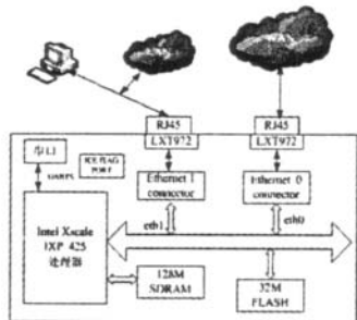
图 1 嵌入式 IPv6 防火墙硬件体系结构
