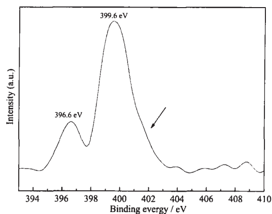
图3 \text{Fe/N-TiO}_2 表面 \text{N1s} XPS图谱
