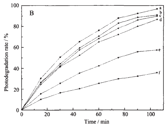
A: Under UV-light B: Under sunlight (a) 0.45% Fe 3+ ; (b) 0.82% Fe 3+ ; (c) 1.14% Fe 3+ ; (d) 0.16% Fe 3+ ; (e) N-TiO 2 ; (f) TiO 2
