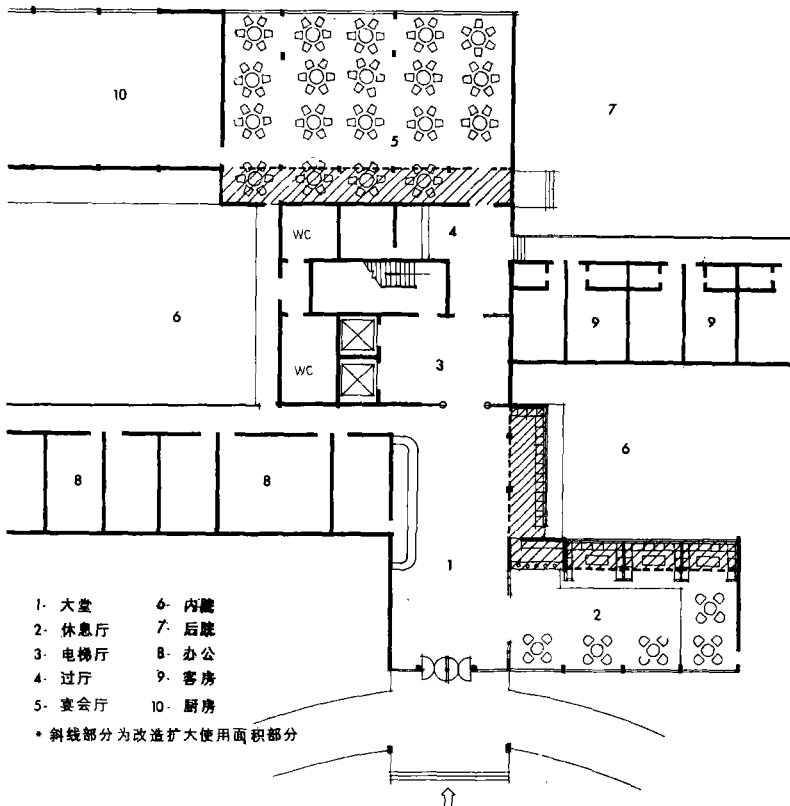
1 宾馆公共部分平面调整
