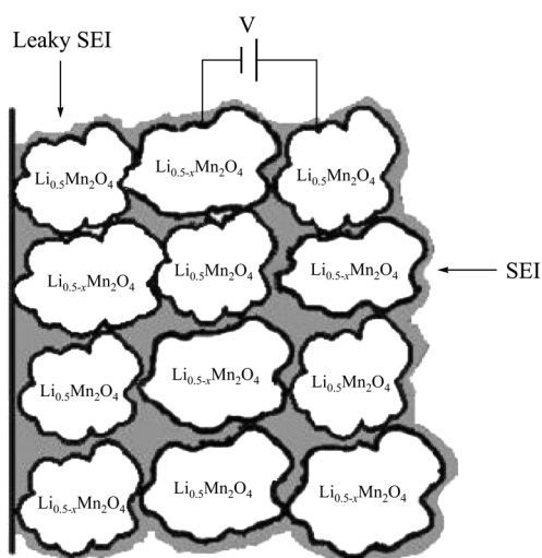
图 13 尖晶石 \text{LiMn}_2\text{O}_4 电极在首次充放电过程中, \text{Li}_{0.5}\text{Mn}_2\text{O}_4/\text{Li}_{0.5-x}\text{Mn}_2\text{O}_4 局域浓差电池模型示意图
