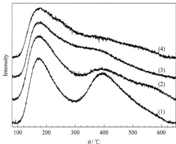
图 5 不同载体及其负载型 Ni 基催化剂的 \text{NH}_3 -TPD 谱
