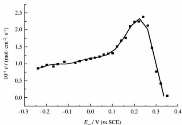
图4 高氯酸介质中 Pt(111)-I 上 EG 解离吸附的平均速率(30 s 区域)随 E_{ad} 的分布
