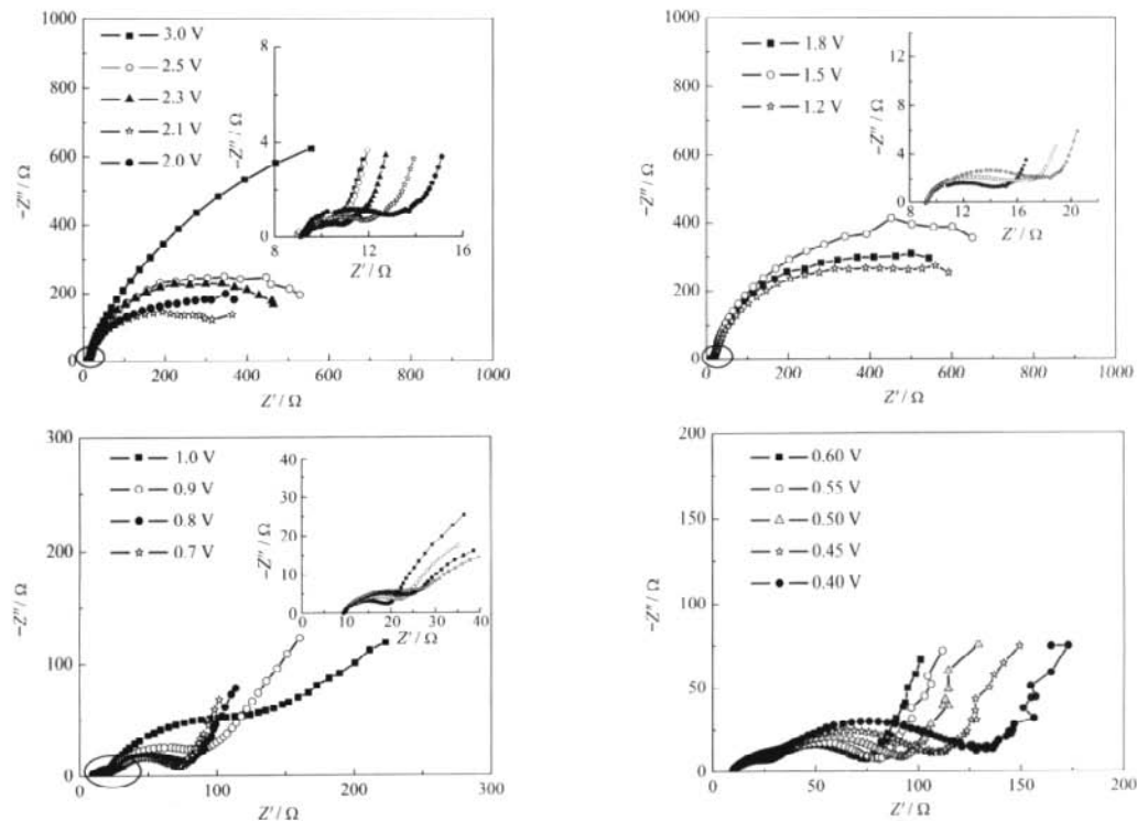
图 3 60 °C 时石墨电极在 1 mol·L -1 LiPF 6 -EC:DEC:DMC+5%VC 电解液中首次阴极极化过程中 Nyquist 图随电极电位(3.0–0.4 V)的变化
