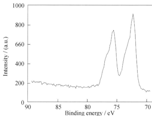
图 4 \text{C}_{60}\text{Pt}(\text{dppp}) \text{Pt}4f_{7/2} 的 XPS 图谱
