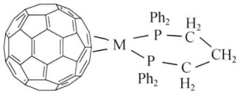
图 5 C 60 Pt(dppp)结构示意图
