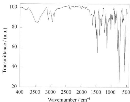
图 3 \text{C}_{60}\text{Pt}(\text{dppp}) 的红外光谱图
