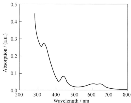
图 2 \text{C}_{60}\text{Pt}(\text{dppp}) 的紫外可见光谱图
