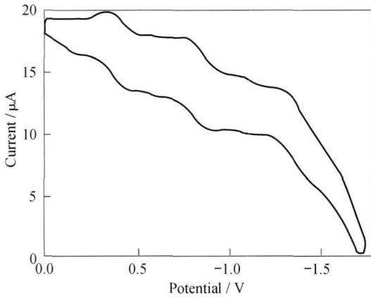
图 6 C 60 Pt(dppp)循环伏安曲线
