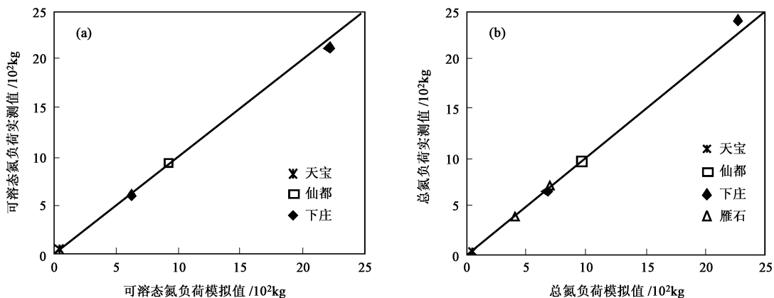
图4 九龙江典型小流域氮输出模拟值与实测值拟合图
