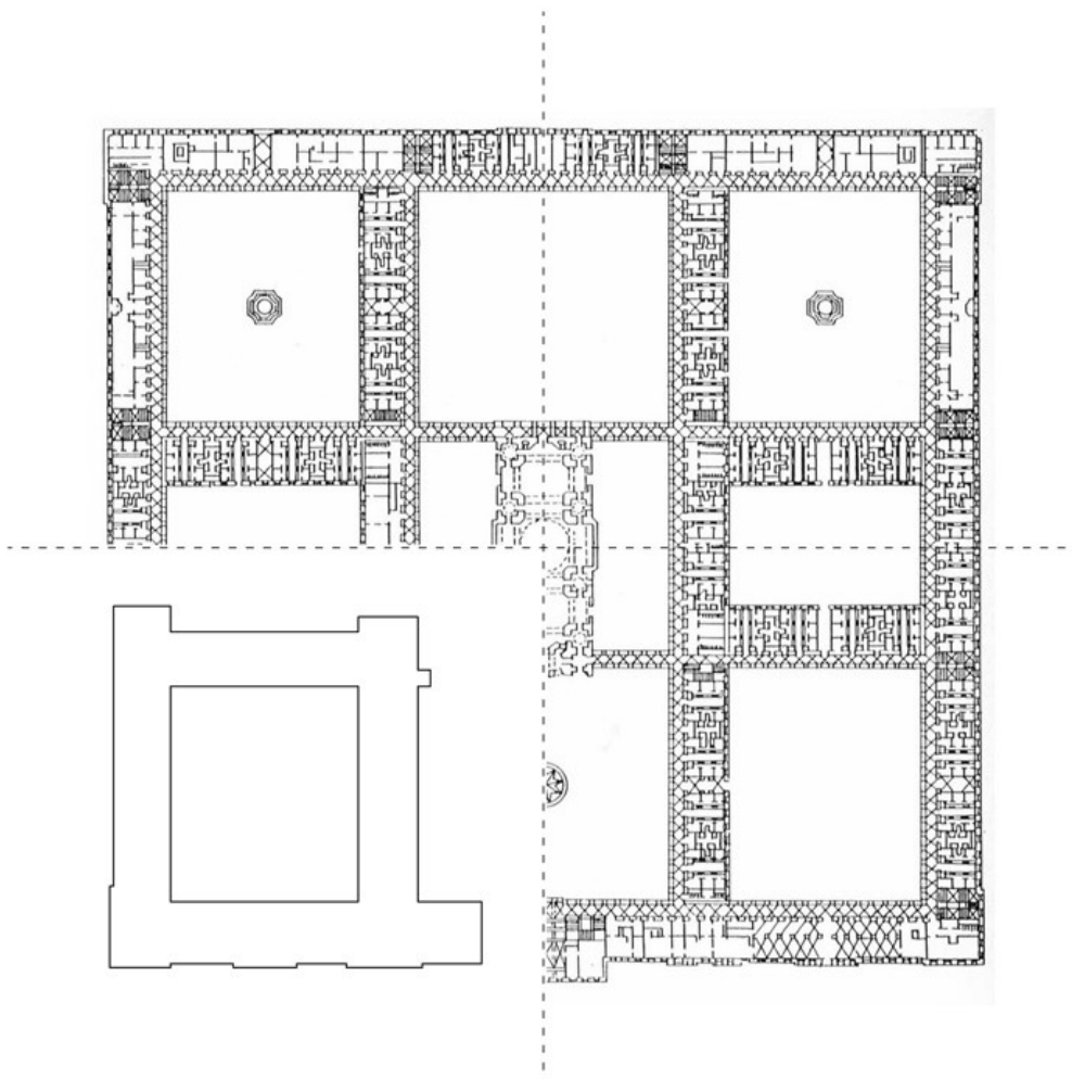
11. Nákres půdorysu pražské invalidovny v původně zamýšleném rozsahu. Vlevo dole je schéma realizované části, představující jeho jednu devítinu 280
