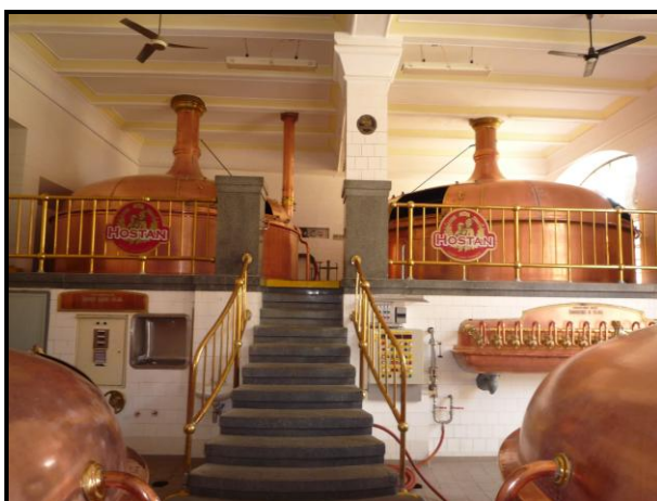
Obr. 35: Vnitřní vybavení varny, měděné pánve z roku 1935.
