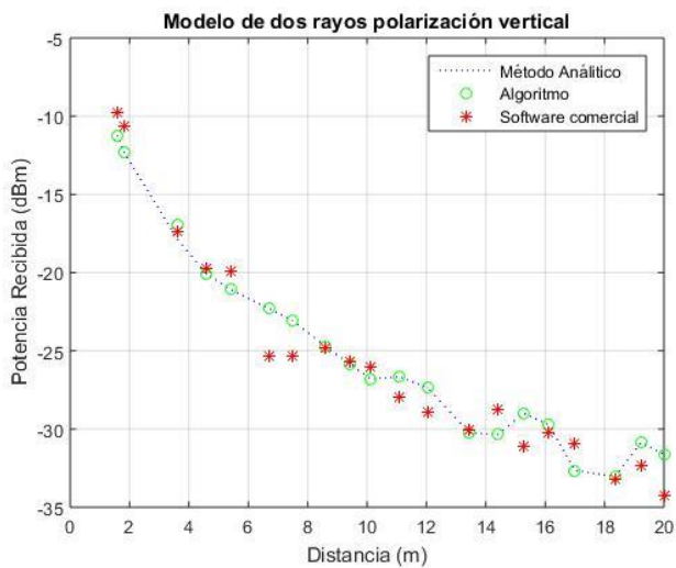
Figura 5: Potencia recibida en el receptor respecto a la distancia en modelo de dos rayos con antena vertical. Fuente: Elaboracion propia.
