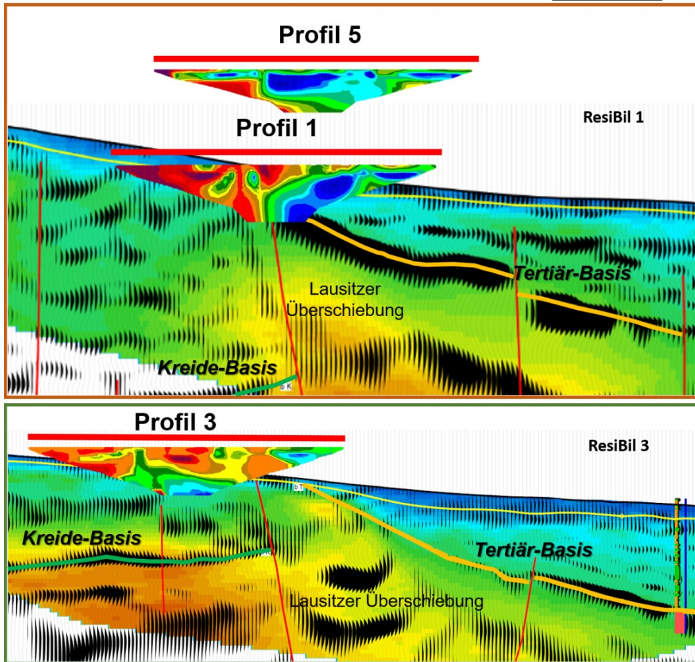
Abb. 33: Erfassung der Lausitzer Überschiebung mit den Seismik-Profilen ResiBil 1 und ResiBil 3 sowie den ERT-Profilen 1, 3 und 5.
