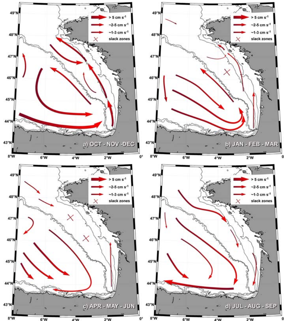
FIG. I.10 – (issue de Charria et al., 2011 : Courants saisonniers à 15m. La largeur des flèches est proportionnelle à l'intensité des courants. Les croix représentent les zones où le courant est très faible
