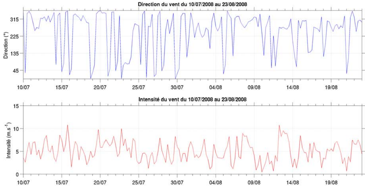
FIG. IV.16 – Vent instantané en ( 44.5^{\circ}\text{N}, 1.5^{\circ}\text{W} ) en 2008 - Données ARPEGE traitées toutes les 6h
