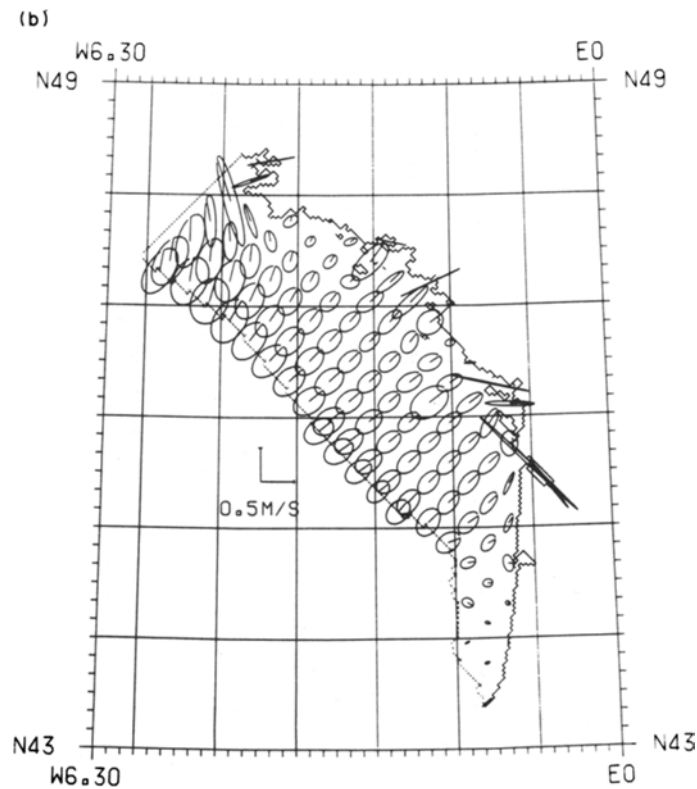
FIG. I.7 – (issue de Le Cann, 1990) : Ellipses de marée M2
