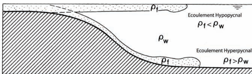
Figure I-21 - Écoulement hyperpycnal et écoulement hypopycnal. \rho_f correspond à la densité de l'écoulement et \rho_w correspond à la densité du fluide ambiant (d'après Mulder et Alexander, 2001)
