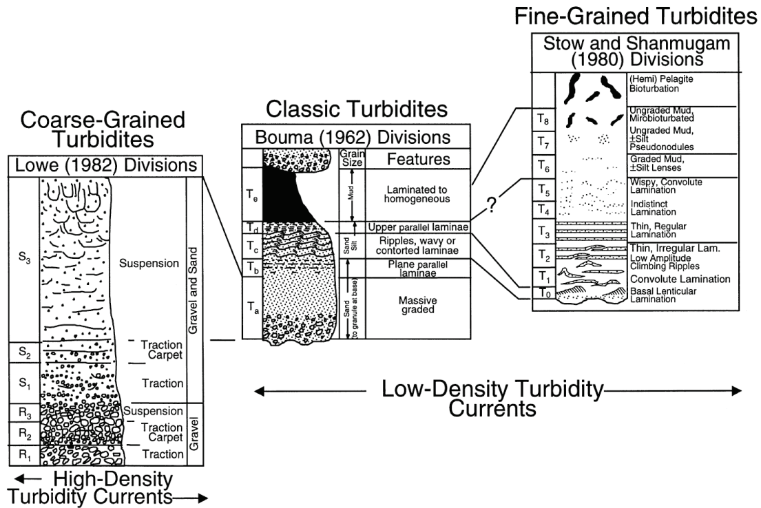
Figure I-20 - Séquences turbiditiques « types » définies par Bouma (1962), Lowe (1982) et Stow et Shanmugam (1980) (d'après Shanmugam, 2000).
