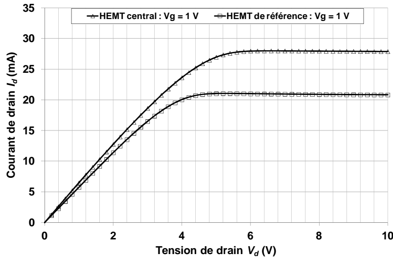
Figure IV.30 : Courbes I_d(V_d) du HEMT de référence et du HEMT central pour V_g = 1 V
