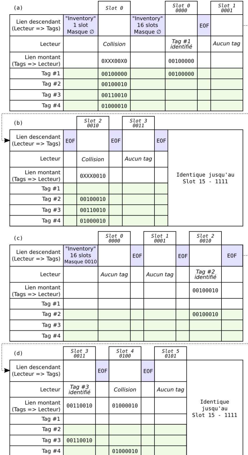
Figure D-3 : Exemple d'exécution de l'algorithme d'anticollision défini dans la norme ISO15693
