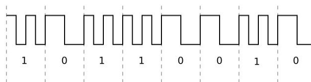
Figure B-7 : Codage « AC »
