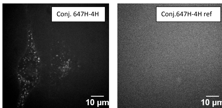
Figure III.14. Clichés de microscopie confocale (x3) réalisés sur des cellules HeLa incubées 2h à 37°C et sous 5% de CO 2 en présence de bio-conjugués 647H-4H et 647H-4H ref à 1 µM (Ex = 635 nm / filtre émission = 725/150 nm).
