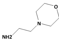
Figure III.5. Structure de la 4-(2-Aminoéthyl)morpholine (AEM) utilisée pour le capping des fonctions ester activé restantes après couplage des chromophores.
