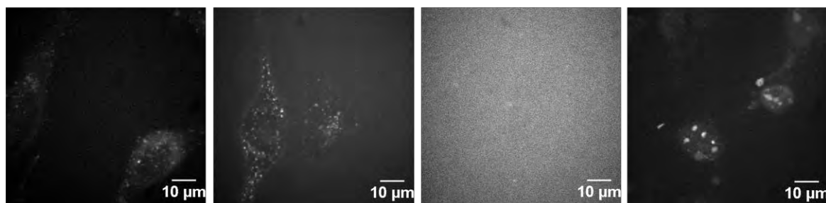
Figure III.12. Clichés de microscopie confocale ( \times 63 ) réalisés sur des cellules HeLa incubées 2h ( 37^{\circ}\text{C} et sous 5% de \text{CO}_2 ) en présence bio-conjugués 20K-4H ( 0,5 \mu\text{M} ), 647H-4H ( 1 \mu\text{M} ) et 33K-9H(LY) ( 1 et 0,5 \mu\text{M} ).
