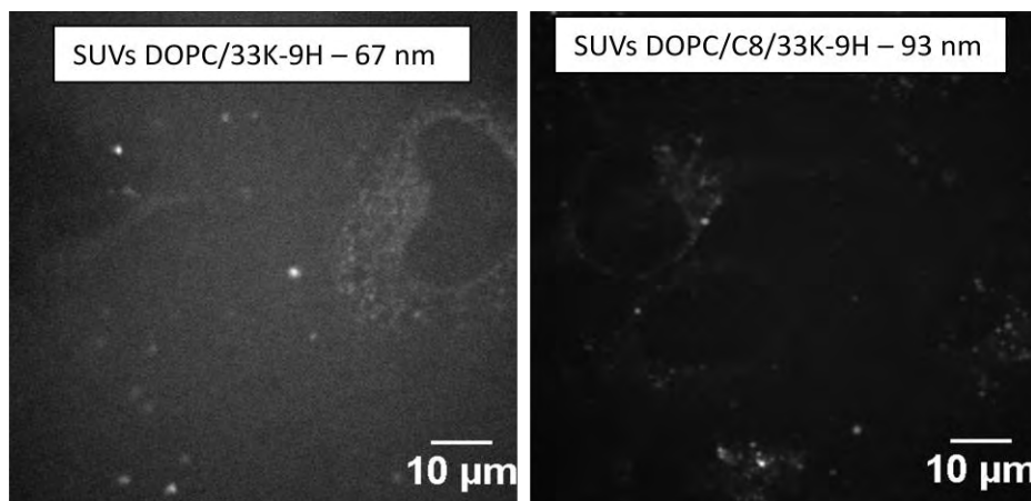
Figure 7-4. Clichés de microscopie confocale de fluorescence ( \times 63 ) des cellules HeLa incubées 2h à 37°C et sous 5% de CO 2 en présence de SUVs DOPC/conjugué 33K-9H (gauche), de SUVs DOPC/C8/conjugué 33K-9H (droite). (Ex = 491 nm / filtre émission = 675/67 nm)
