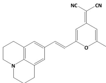
Figure II.5. Exemple d'un chromophore basé sur une structure de type pyrane : le DCM2 (4-(dicyanométhylène)-2-méthyl-6-[4-diméthylaminostyril]-4H-pyran]).
