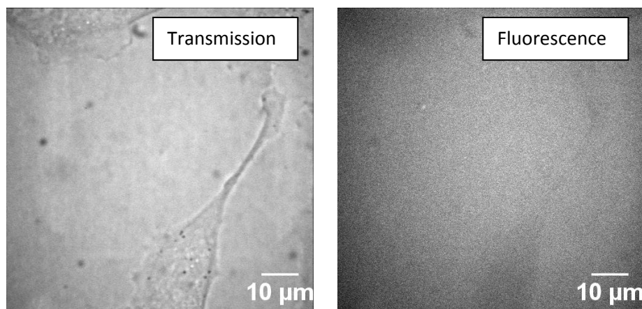
Figure III.17. Clichés de microscopie confocale ( \times 63 ) de cellules HeLa incubées en présence de LUVs fluorescentes (97 nm) pendant 30 min ( 37^{\circ}\text{C} et sous 5% de \text{CO}_2 ). (Ex = 491 nm / filtre émission = 675/67 nm)
