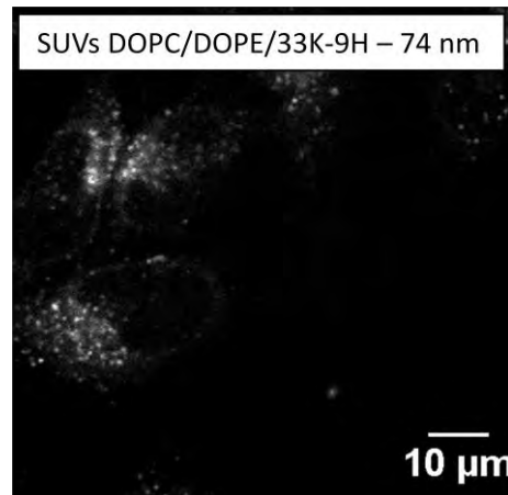
Figure 7-3. Clichés de microscopie confocale de fluorescence ( \times 63 ) des cellules HeLa incubées 2h à 37°C et sous 5% de CO 2 en présence de SUVs DOPC/DOPE/33K-9H. (Ex = 491 nm / filtre émission = 675/67 nm)
