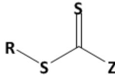
Figure 2. Structure générale des agents de transfert RAFT.
