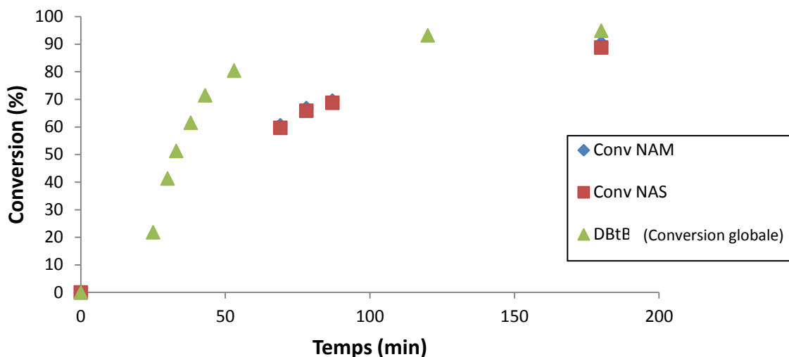
Figure III.5. Cinétique de polymérisation des monomères NAM et NAS par voie RAFT. ATC : ATC-DPPEHA ; [Monomères] = 2 M ; Amorceur AIBN ; [ATC]_0 / [AIBN]_0 : 5 ; T = 80^\circ C ; dioxane.
