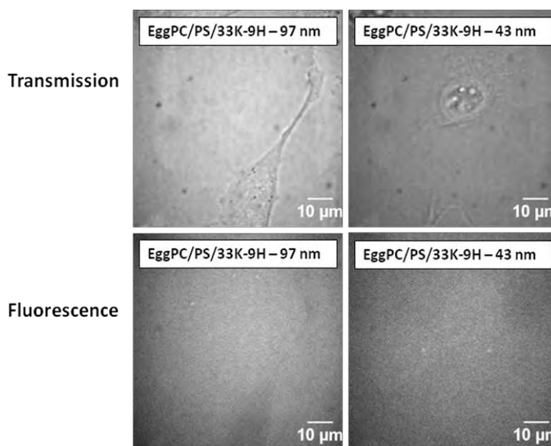
Figure III.18. Clichés de microscopie confocale (Transmission et Fluorescence) ( \times 63 ) des cellules Hela incubées 2h (37°C et sous 5% de CO 2 ) en présence de SUVs et de LUVs fluorescentes. (Ex = 491 nm / filtre émission = 675/67 nm)
