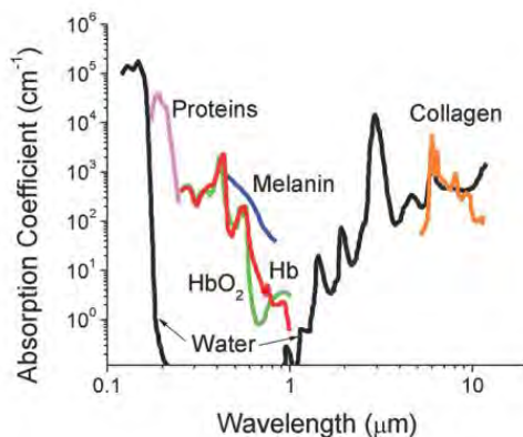
Figure II.1. Graphique représentant l'absorption de divers tissus et composants sanguins pour des longueurs d'ondes comprises entre 100 nm et 10 \mu\text{m} 6 .
