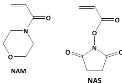
Figure 1.3. Structure du monomère NAM conduisant à des polymères hydrophiles et biocompatibles et du monomère réactif NAS.
