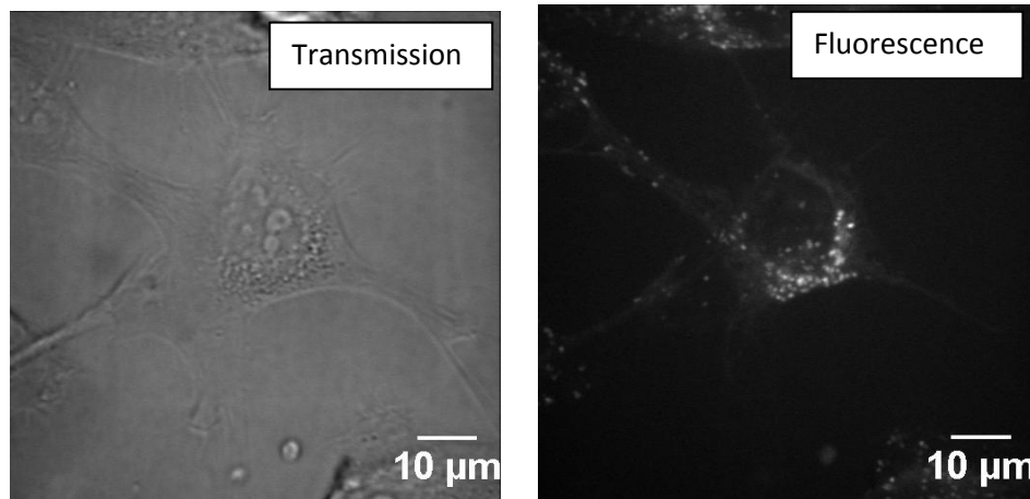
Figure III.1. Clichés de microscopie ( \times 63 ) d'une même cellule Hela après incubation 1h30 à 37°C et sous 5% de \text{CO}_2 en présence de bio-conjugué 33K-9H à 1 \mu\text{M} (Ex = 491 nm / filtre émission = 675/67 nm).
