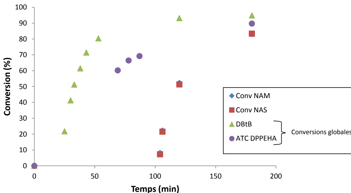
Figure III.7. Cinétique de polymérisation des monomères NAM et NAS par voie RAFT. ATC : ATC-DPPE ; [Monomères] = 2 M ; Amorceur AIBN ; [ATC] 0 / [AIBN] 0 : 5 ; T = 80°C ; dioxane.
