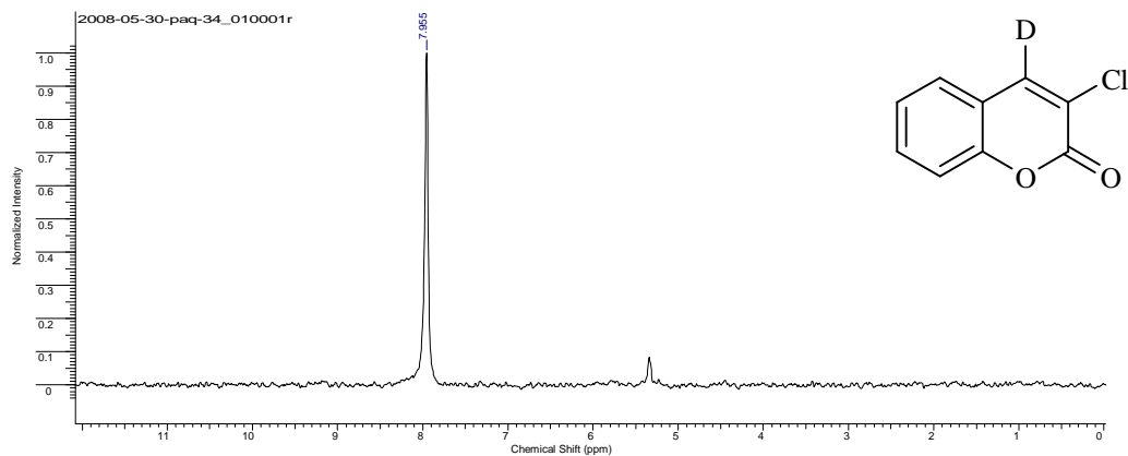
^2\text{H} NMR ( \text{CH}_2\text{Cl}_2 ) of 3-Chloro-2 H -chromen-2-one-d-1 (331)
