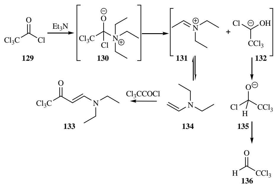
Scheme 2.19. \text{Cl}_3\text{CCOCHCHNEt}_2 formation.
