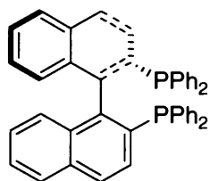
Figure 1.4 BINAP
