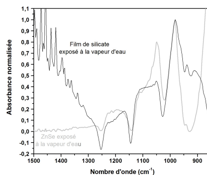
FIGURE 7.13 – Comparaison du spectre du film de silicate après exposition à la vapeur d'eau (en noir) avec celui du ZnSe après exposition (en gris) . Les deux spectres sont normalisés à leur pic de plus forte absorbance dans la gamme [1300\text{ cm}^{-1} - 850\text{ cm}^{-1}] .
