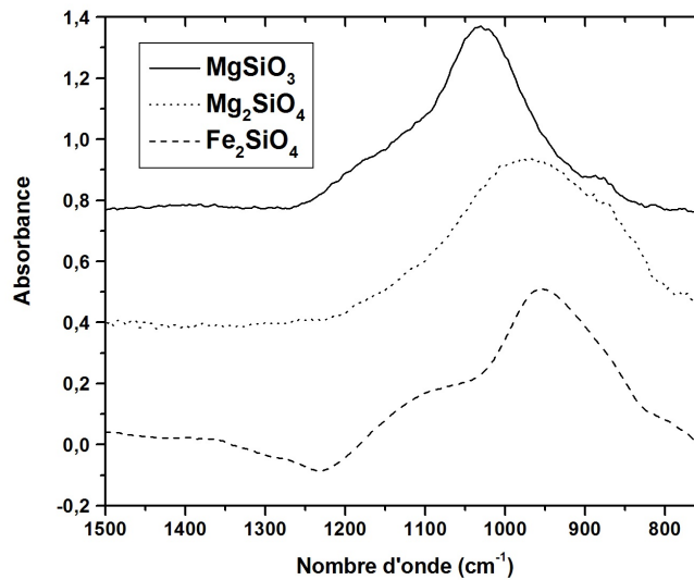
FIGURE A.5 – Spectres IR dans la gamme 1500\text{ cm}^{-1} ( \sim 6.7\ \mu\text{m} ) à 750\text{ cm}^{-1} ( \sim 13.3\ \mu\text{m} ) de films amorphes de compositions d’énstatite ( \text{MgSiO}_3 ), forstérite ( \text{Mg}_2\text{SiO}_4 ) et fayalite ( \text{Fe}_2\text{SiO}_4 ). Les spectres ont été normalisés à leur plus haut pic et décalés verticalement pour plus de clarté.
