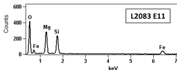
FIGURE 4.12 – Spectre EDX de l'IDP L2083 E11 obtenu avec une tension de 15 kV.
