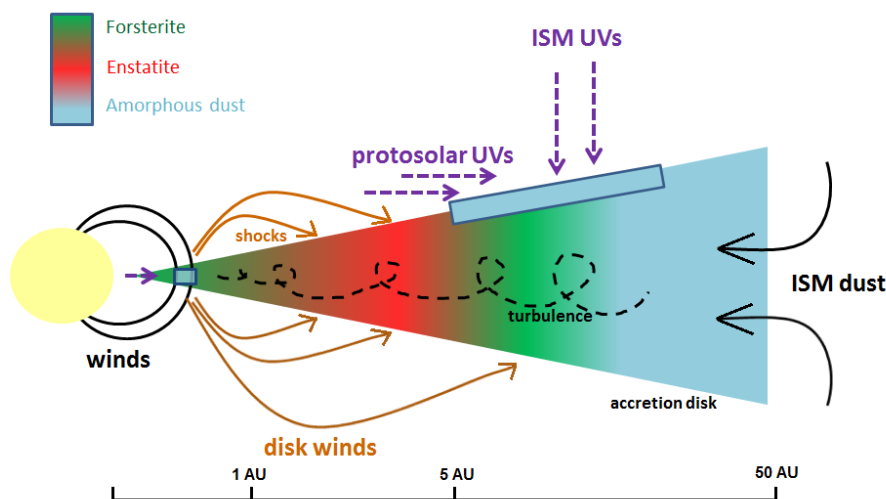
FIGURE 1.4 – Illustration des différents processus ayant lieu dans le disque protoplanétaire à partir des modèles de Wooden (2008); Aléon (2008); Krot et al. (2009).
