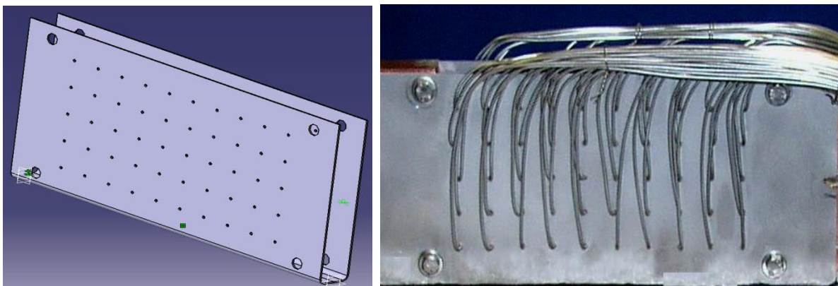
Figure III.11. Creuset en acier inoxydable avec le faisceau d'acquisition de la température qui comporte 66 thermocouples de type K soudés par laser : 50 sur la paroi latérale (vue de face) et 16 sur l'autre paroi latérale.
