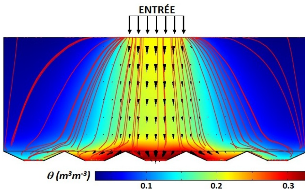
Figure IV-18 : Distribution de la teneur volumique en eau, \theta ( \text{m}^3 \text{m}^{-3} ), champ vectoriel de flux darcien (flèches) et lignes de courant (courbes) en régime stationnaire pour le PROF1 et la vitesse 1.21 \times 10^{-5} \text{ m s}^{-1} .
