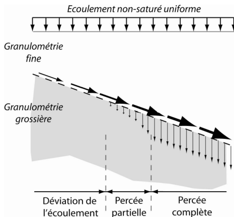
Figure I-8 : Écoulement préférentiel dû aux flux latéraux, d'après Heilig et al. (Heilig et al., 2003).
