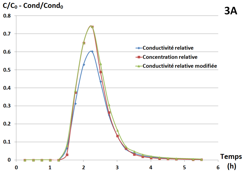
Courbes d'élution de la sortie 3A par les deux méthodes d'analyse.
