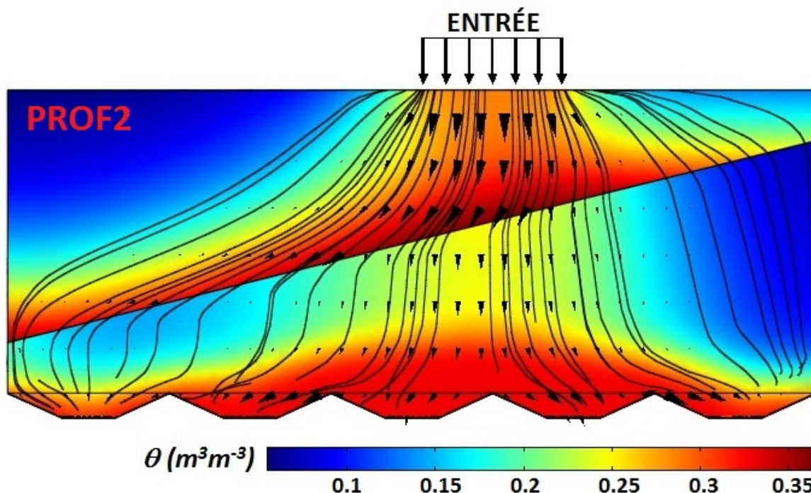
Figure IV-10 : Distribution de la teneur volumique en eau, \theta (m^3 m^{-3}) , champ vectoriel de flux darcien (flèches) et lignes de courants (courbes) en régime stationnaire pour l'essai E2.
