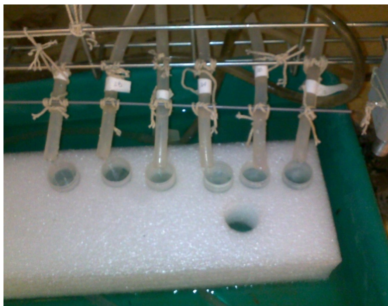
Figure II-25 : Collecte des échantillons.
