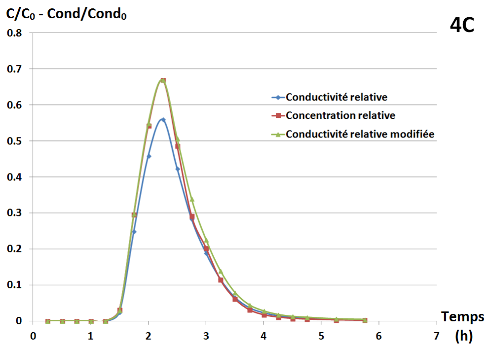
Courbes d'élution de la sortie 4C par les deux méthodes d'analyse.
