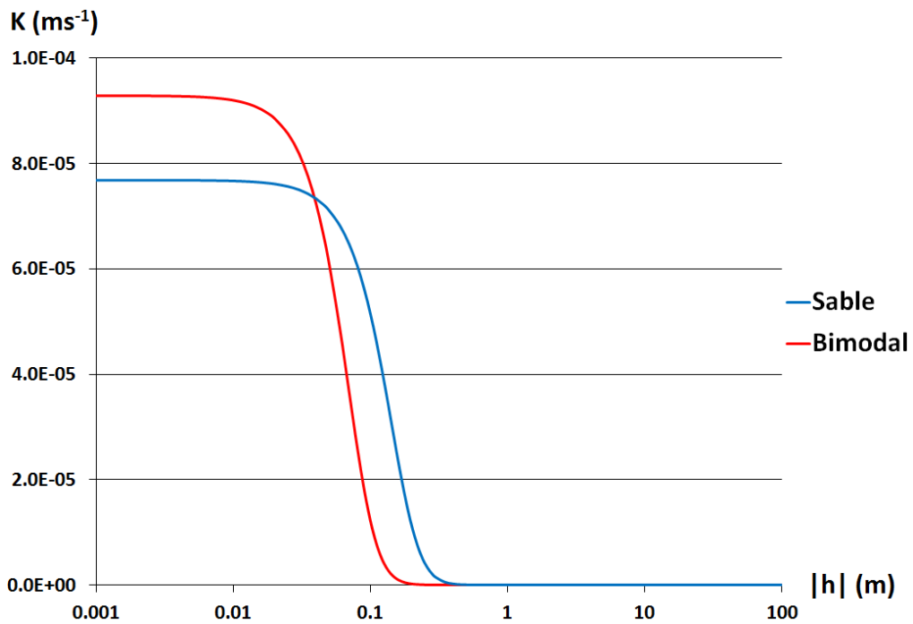
Figure II-7: Courbes de conductivité hydraulique K(h) des matériaux utilisés caractérisées par le modèle de van Genuchten-Mualem.
