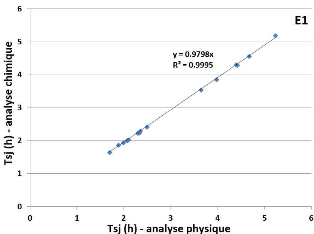
Figure III-8 : Temps de séjour du soluté de quinze courbes d'élution mesuré par les deux méthodes : conductivité électrique et analyse chimique.
