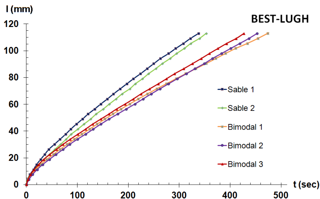
Figure II-4 : Infiltration cumulée des essais Beerkan en lysimètre LUGH pour le sable et le mélange bimodal.
