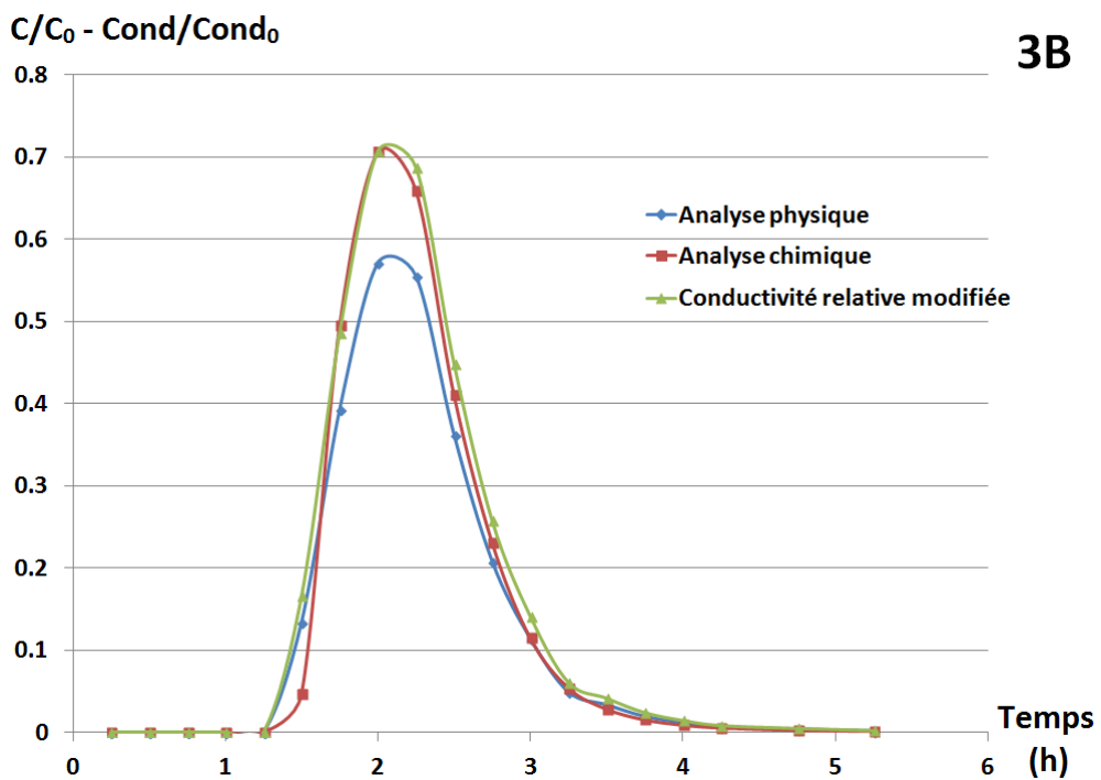
Courbes d'élution de la sortie 3B par les deux méthodes d'analyse.
