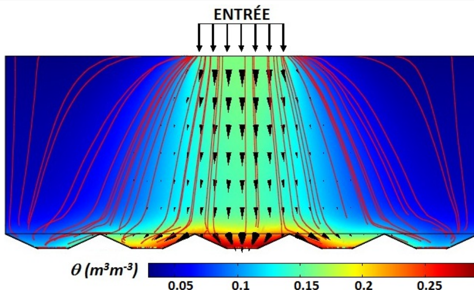
Figure IV-19 : Distribution de la teneur volumique en eau, \theta ( \text{m}^3 \text{m}^{-3} ), champ vectoriel de flux darcien (flèches) et lignes de courant (courbes) en régime stationnaire pour le PROF1 et la vitesse 3.62\text{e-}6 \text{ m s}^{-1} .
