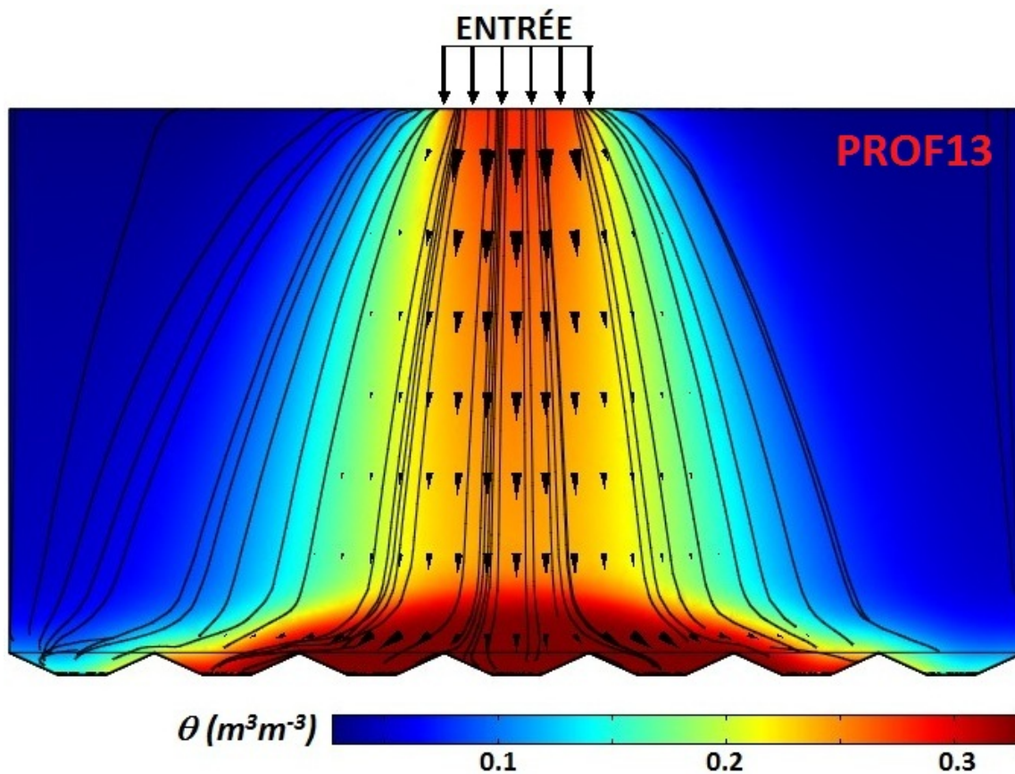
Figure IV-15 : Distribution de la teneur volumique en eau, \theta (m^3 m^{-3}) , champ vectoriel de flux darcien (flèches) et lignes de courant (courbes) en régime stationnaire pour le profil PROF13 (combinaison du doublement de la hauteur de sol et de l'augmentation latérale de deux sorties supplémentaires).
