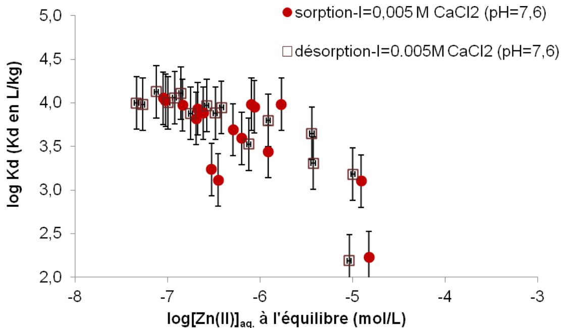
Figure III.5 : Comparaison des isothermes d'adsorption et de désorption de Zn(II) mesurées avec le sol RDB-Z en milieu CaCl_2 5 \times 10^{-3} mol/L à pH=7,6 \pm 0,2 .
