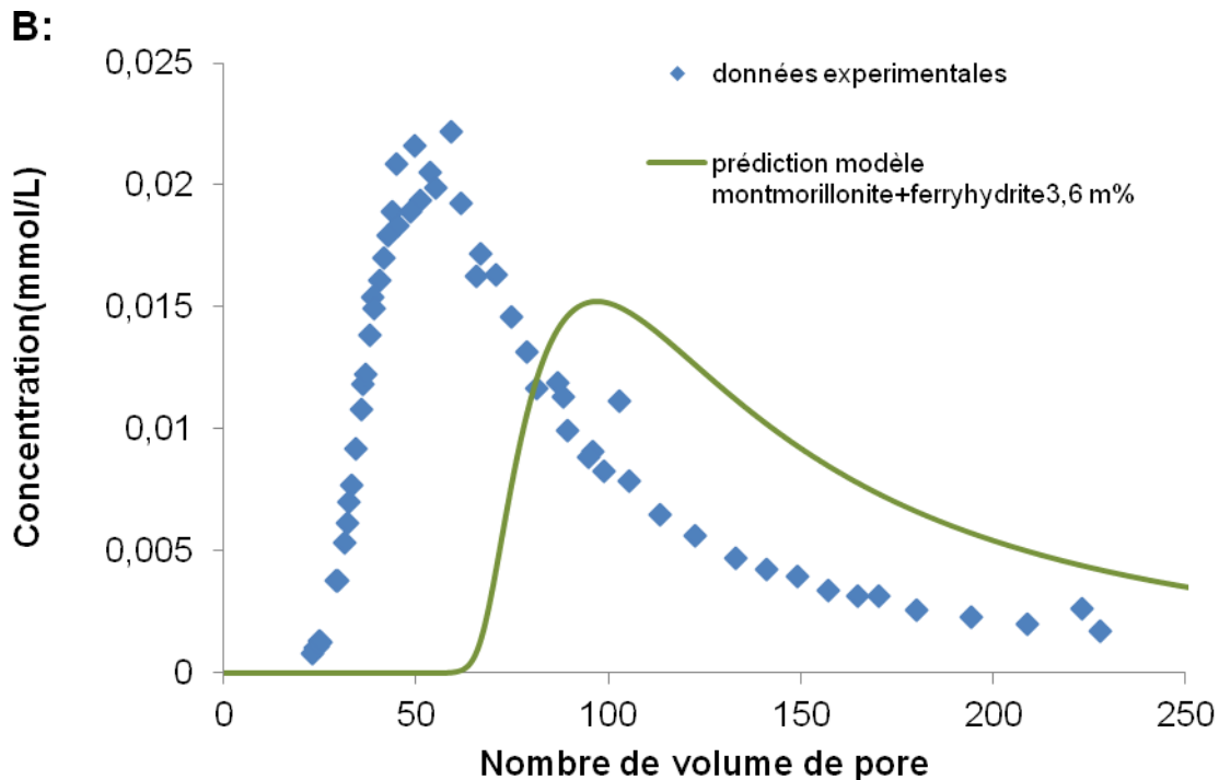
Figure III.14 : Courbes de percée du Zn(II) obtenue avec 0,005 M CaCl 2 comme électrolyte. Comparaison entre données expérimentales et données prédites par le modèle d'adsorption basé sur un assemblage de la ferryhydrite 3,6m% et de la montmorillonite avec les coefficients de sélectivité K_{2H/Zn}^{si} obtenus respectivement par interprétation des données expérimentales de Baeyens and Bradbury en milieu Na (A) et en milieu Ca (B).
