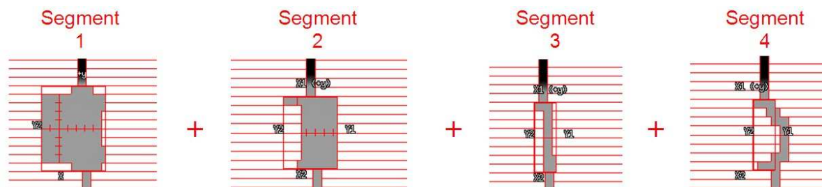
Figure 4 : Exemple de faisceau possédant 4 segments en technique de RCMI type « Step and Shoot ».
