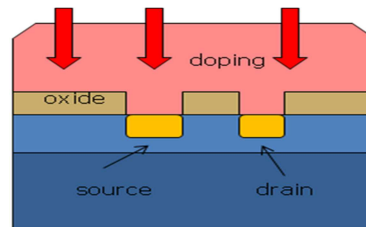
Figure 63 : Implantation ionique pour formation des zones source et drain
