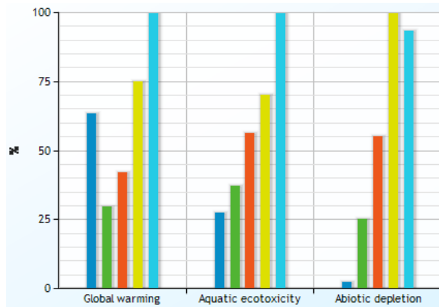
■ Gravure Salicide Protect ■ Gravure Floating Gate ■ Gravure Self Aligned ■ Gravure Gate ■ Gravure STI
