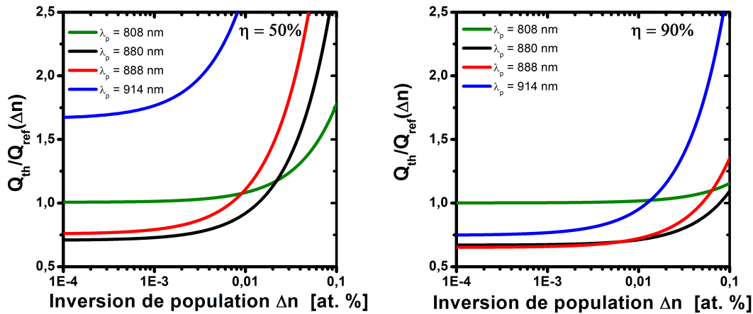
FIGURE 7.11 – Évolution de la charge thermique avec l'inversion de population pour différentes longueurs d'onde de pompe \lambda_p et taux d'extraction \eta .
