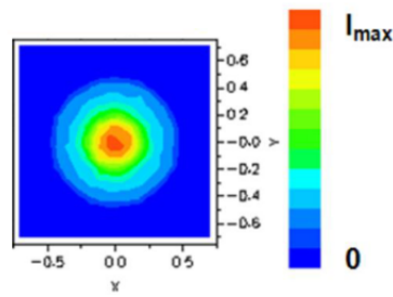
FIGURE 2.6 – Distribution d'intensité calculée dans la partie guidée (à 40\text{ mm} de la face d'entrée) avec le logiciel Apilux. Fibre cristalline de 1\text{ mm} de diamètre. Faisceau avec une ouverture numérique incidente de 0,22 et 400\ \mu\text{m} de diamètre au col. (Extrait de la thèse de Damien Sangla) [Sangla 09a]
