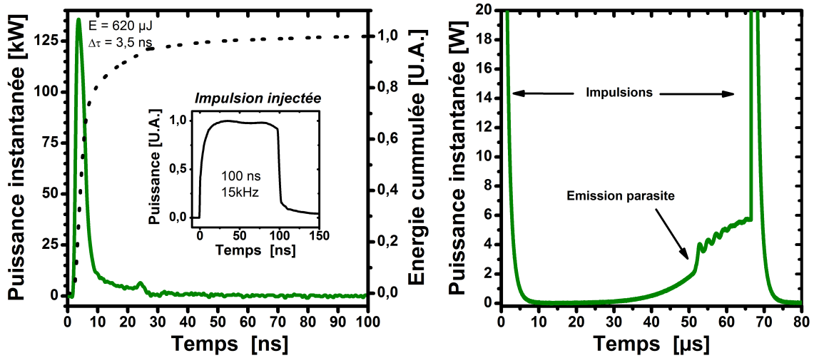
FIGURE 8.12 – Puissance de sortie en fonction du temps. Paramètres du signal en entrée : (Puissance moyenne : 350 \mu\text{W} , Fréquence de répétition : 15 \text{ kHz} , Durée : 100 \text{ ns} ). Paramètres du signal en sortie : (Puissance moyenne : 9,2 \text{ W} + 1,3 \text{ W} d'émission parasite, Fréquence de répétition : 15 \text{ kHz} , Durée : 3,5 \text{ ns} ).
