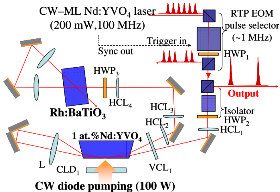
FIGURE 8.1 – Amplificateur Nd:YVO 4 en configuration à incidence rasante [Nawata 09].
