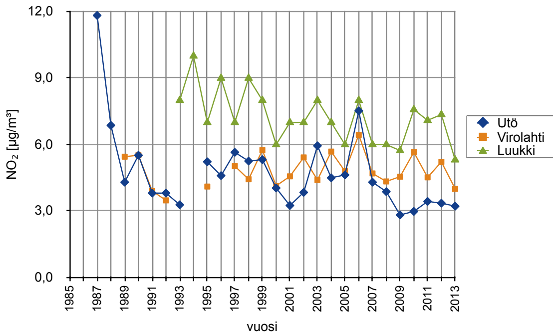
Kuva 17. Typpidioksidin pitoisuus ( \mu\text{g}/\text{m}^3 ) ilmassa, vuosikeskiarvot Utön, Virolahden ja Espoon Luukin mittausasemilla vuosina 1985–2013. (Niemi 2009, Salmi 2009, Ilmanlaatuportaali 2015). Figur 17. Halten av kvävedioxid ( \mu\text{g}/\text{m}^3 ) i luften, årsmedeltalet vid mätningstationer i Utö, Vederlax och Luk åren 1985–2013 (Niemi 2009, Salmi 2009, Ilmanlaatuportaali 2015).
