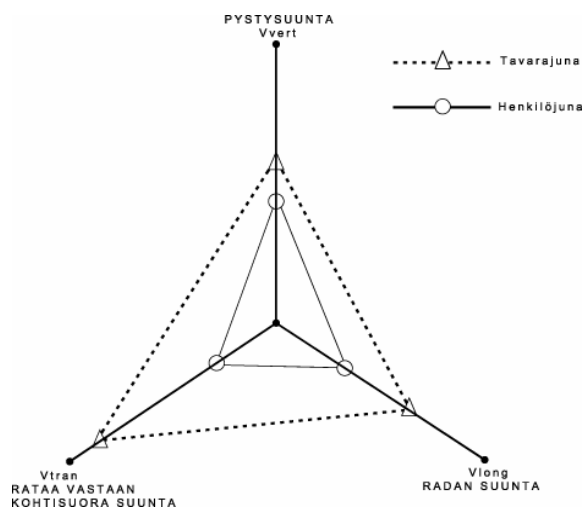
Kuva 13. Esimerkki kolmikomponenttimittauksen tuloksista graafisesti esitettynä / lähde: 18, s.10 mukailen /.
