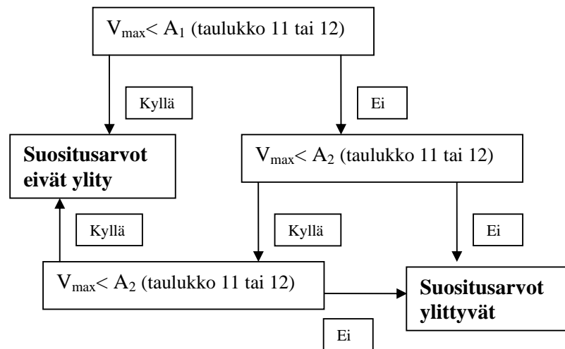
Kuva 22. Suositusarvojen ylittymisen kriteerit Hollannin normin mukaan / 21, s. 24. /
