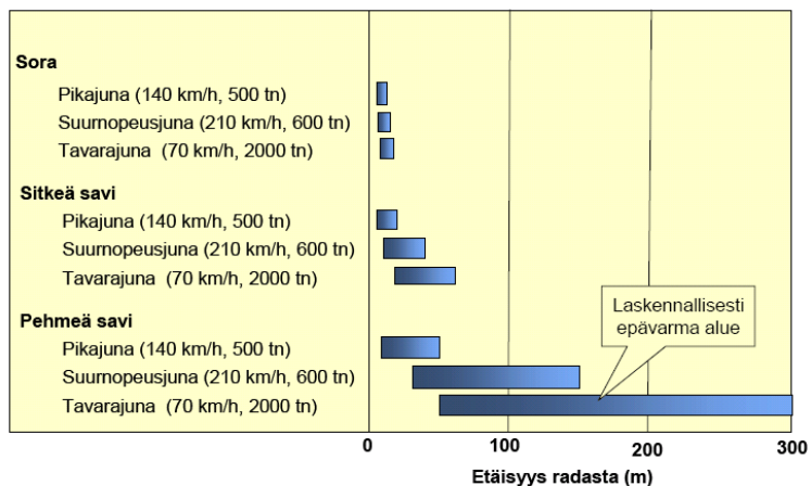
Kuva 11. Arvio etäisyydestä eri maalajeilla, jolloin junista aiheutuva tärinä voi olla haitallinen. Varjostetut alueet ovat laskennallisesti epävarmaa aluetta. / 1. s. 15. /
