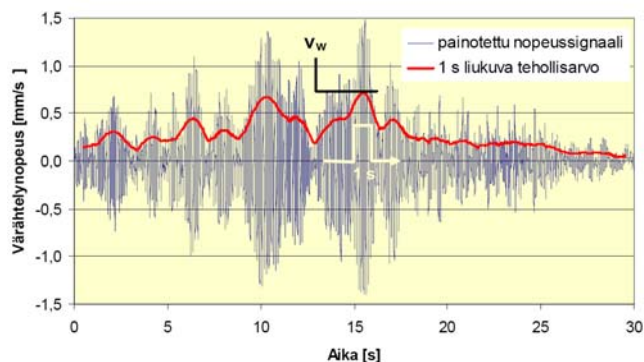
Kuva 14. Suurimman tehollisarvon v_w määrittäminen painotetusta nopeussignaalista 1 sekunnin liukuvan tehollisarvon avulla / 1, s. 20. /
