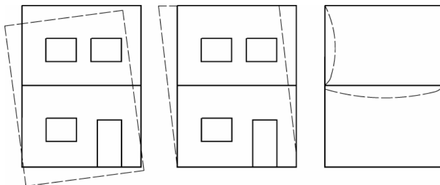
Kuva 6. Esimerkkejä rakennuksen eri värähtelymuodoista / 1, s.19 /.
