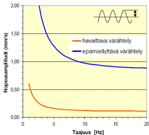
Kuva 9. Ihmisen herkkyys värähtelylle, kun värähtely esitetään värähtelynopeuden avulla / 1, s.13. /
