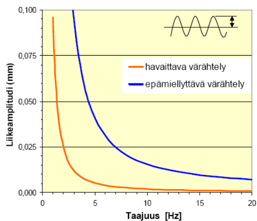
Kuva 8. Ihmisen herkkyyys värähtelylle, kun värähtely esitetään liikkeen avulla. / 1, s.13. /
