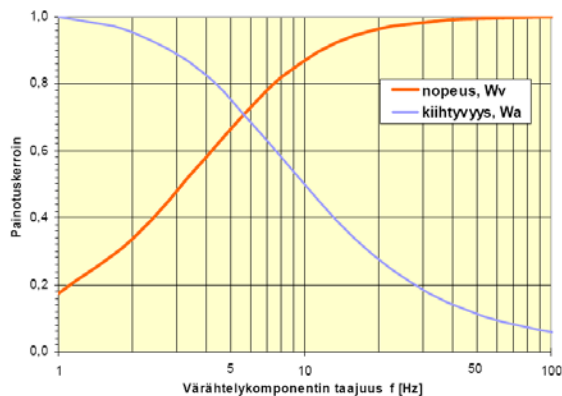
Kuva 15. Värähtelykomponenttien painotuskertoimen nopeus- ja kiihtyvyyssignaaleille. / 1, s.21. /
