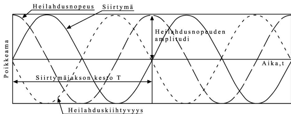
Kuva 2. Harmonisen värähtelyn siirtymä, heilahdusnopeus ja heilahduskihtyvyys ajan suhteen. Kuvaajat ovat samanmuotoisia, mutta eri vaiheissa. / 7, s.5. /
