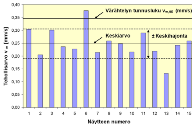
Kuva 17. Periaatekuva värähtelyn tunnusluvun määrittämisestä / 1, s. 24 /.
