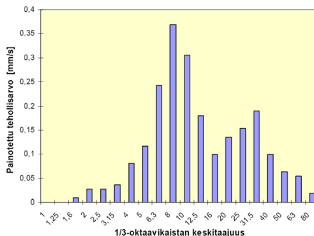
Kuva 16. Värähtelysignaalin painotetut tehollisarvot W_{v,i} v_i kolmannesoktaaveittain / 1, s. 22 /.
