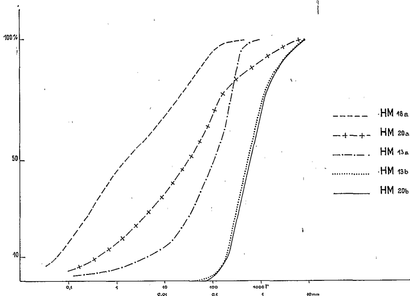
Fig 3 - Dépôts de remblaiement : courbes granulométriques d'échantillons caractéristiques
