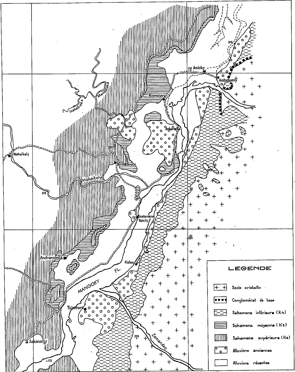
Fig. 1 ESQUISSE GÉOLOGIQUE DE LA MOYENNE VALLÉE DU MANGOKY
