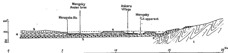
Fig. 2 _ Coupe de la vallée du Mangoky dans la dépression périphérique du massif ancien
