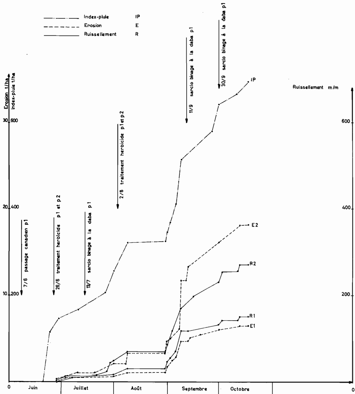
Graphique n° 9 Index-pluie, Erosion et Ruissellement cumulés en fonction du temps. parcelles 1 et 2
