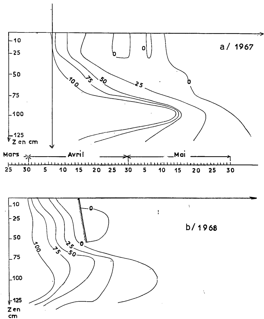
Fig. 2 - Etude de la dé-saturation du sol sous Eucalyptus camaldulensis à l'aide de secondes de Bouyoucos.
