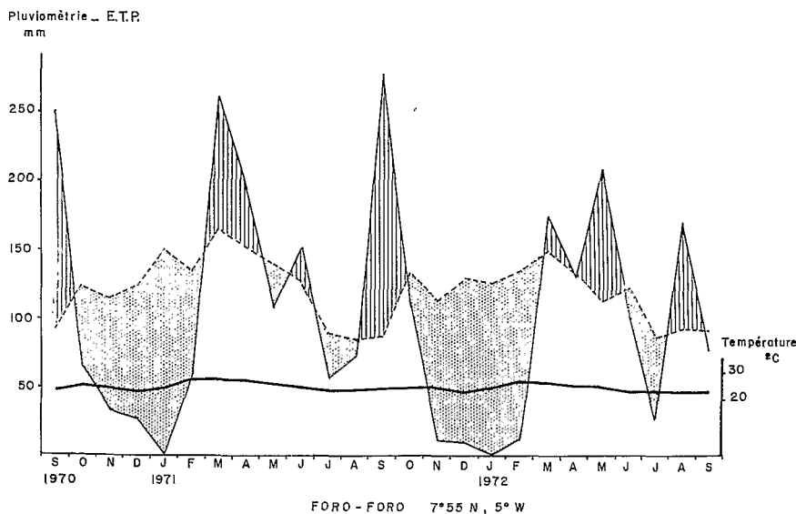
Fig. 1. — Données météorologiques enregistrées au Foro-Foro (7°55 N, 5° W) au cours de la période septembre 1970- septembre 1972. Courbe des températures moyennes (remarquer les deux minimums annuels: juillet, petite saison sèche et décembre, grande saison sèche avec Harmattan), courbe de pluviométrie et courbe d'évapo-transpiration potentielle, calculée selon la formule de TURCK. Les surfaces pointillées représentent les périodes de déficit hydrique, les surfaces hachurées, les périodes où le bilan hydrique est excédentaire. Voir également la figure 4.
