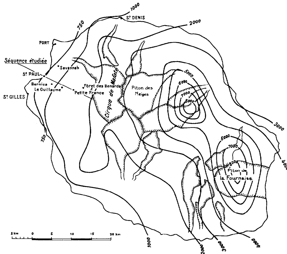
FIG. 1. — Carte de situation et de pluviométrie.
