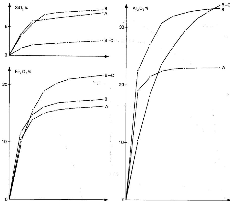
FIG. 8c. — Extraction des produits amorphes du profil RZ 8 (type III).
