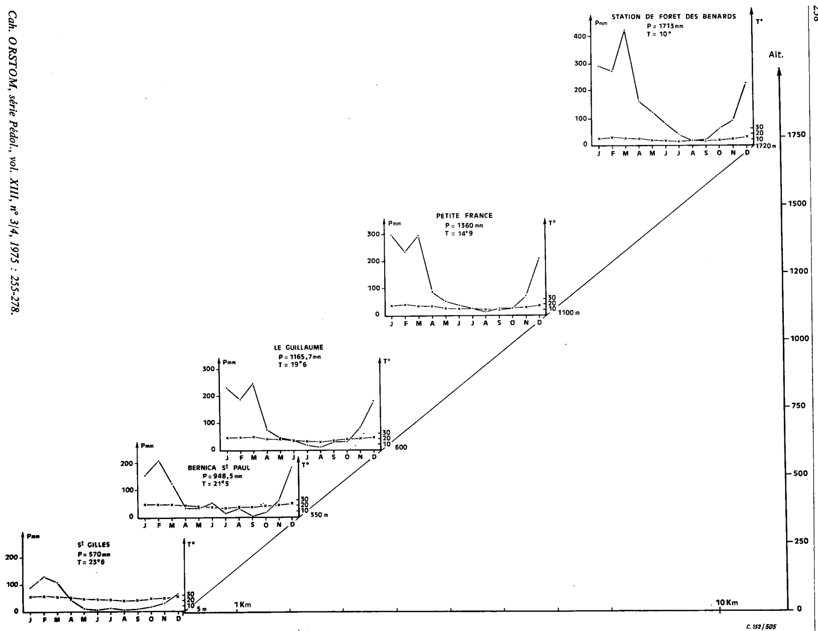
FIG. 2. — Pluviosité et températures en fonction de l'altitude.
