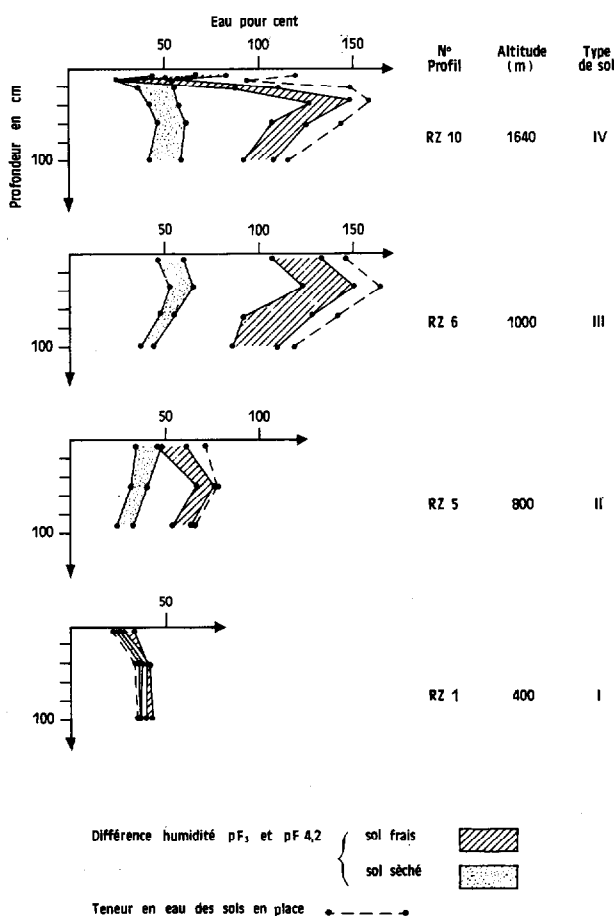
FIG. 4. — Teneurs en eau en % de sol séché à 150°.
