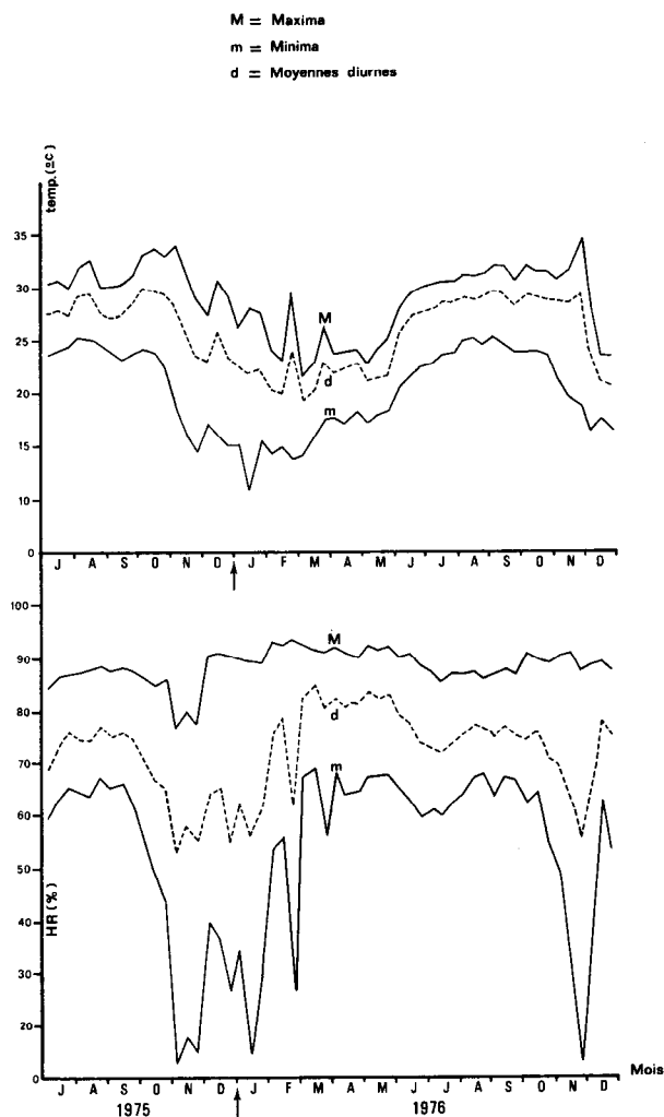
Fig. 2. — Moyennes décadaires des températures et de l'humidité relative (HR) atmosphériques.
