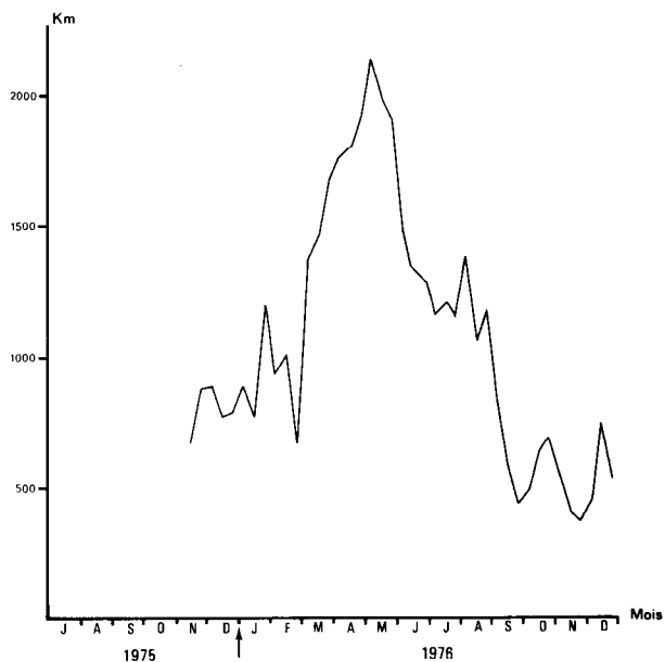
Fig. 1. — Variations saisonnières des distances parcourues par le vent (valeurs cumulées en km par décennie).
