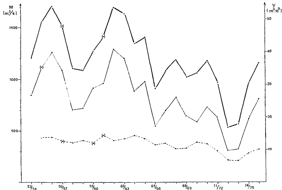
Fig. 2. --- Variations interannuelles des modules ( M , m^3/s ) et des volumes totaux écoulés ( V , 10^3 m^3/s ) en amont du confluent : Logone-Birni (---) et Mailao (—), et après le confluent : N'Djamena (—) de 1953 à 1976.
