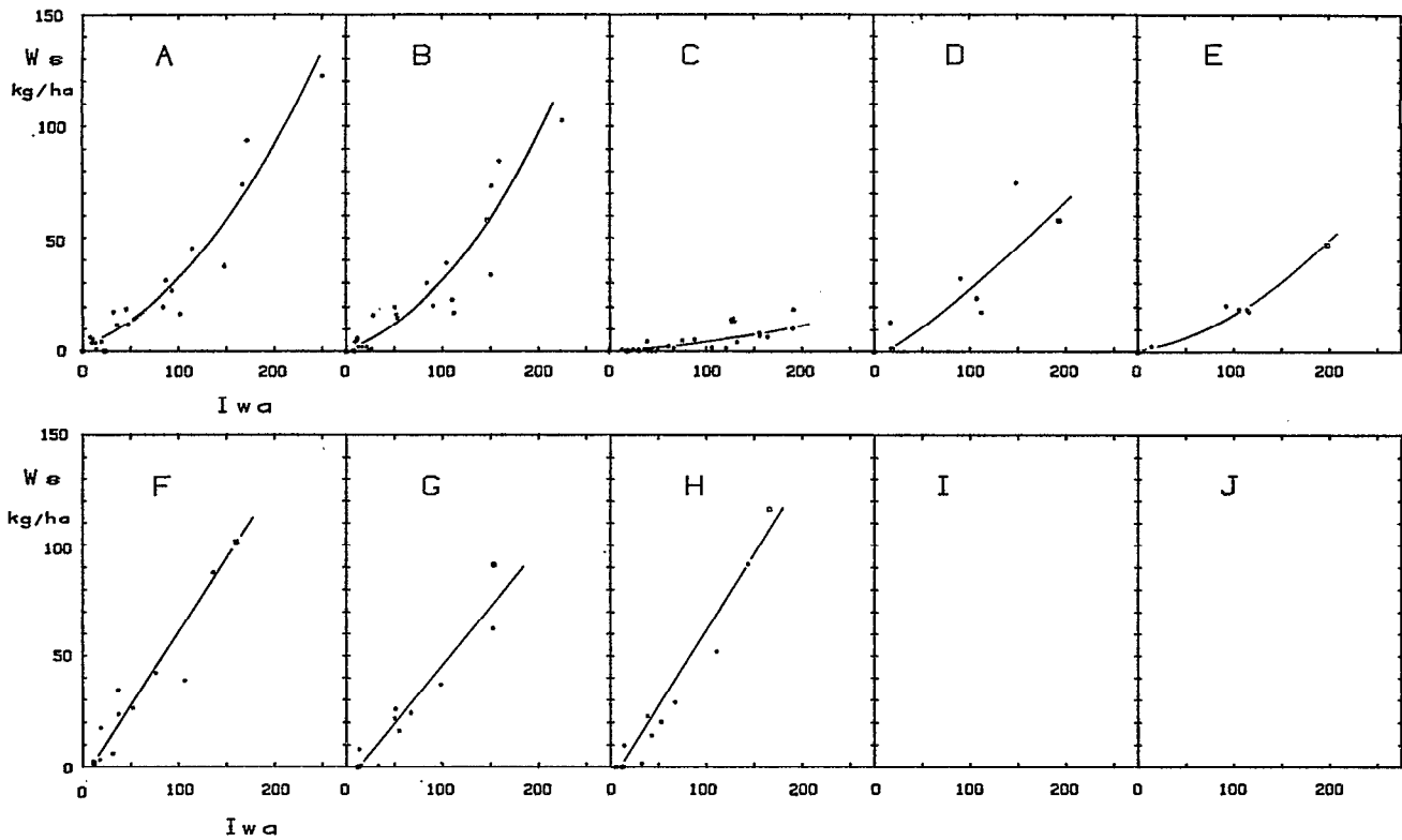
Fig. 7 A. — Ecérex 1977-1978, mensuel. Corrélations entre les quantités de matières en suspension (kg/ha) exportées mensuellement des bassins versants et la somme mensuelle des indices de Wischmeyer (RUSA) des averses ayant provoqué le ruissellement. Les carrés... (idem fig. 1 A)
