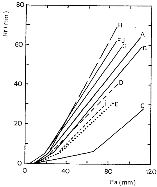
Fig. 8. — Ecérex 1977-1978. Corrélation entre la lame ruisselée à chaque crue et la hauteur de l'averse correspondante. Les courbes définies pour les différents bassins sur la figure 1 A ont été regroupées pour comparaison sur ce même graphique
