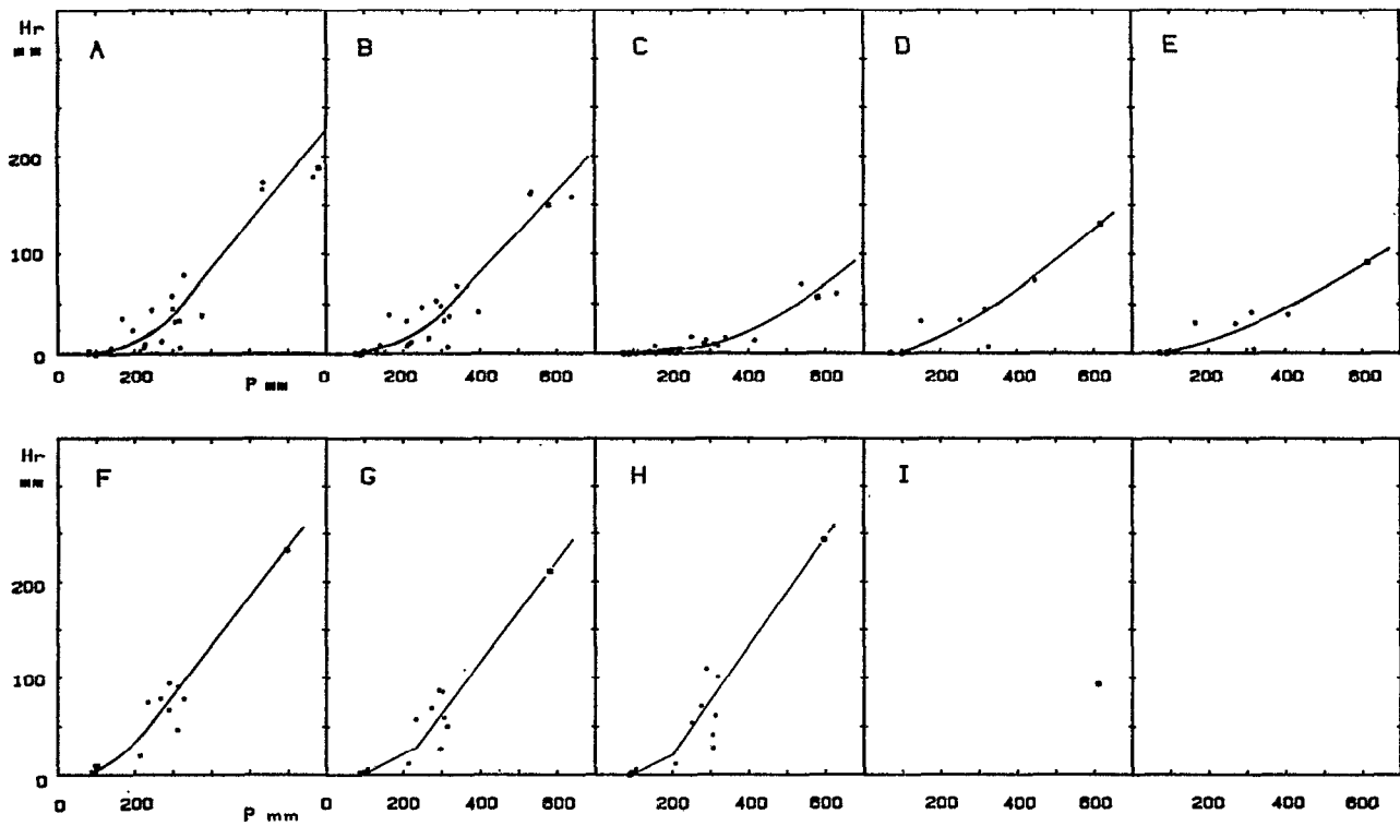
Fig. 3 A. — Ecérex 1977-1978, mensuel. Corrélations entre la lame ruisselée mensuelle (mm) et la hauteur de pluie mensuelle (mm) sur les bassins versants A à I. Les carrés clairs... (idem fig. 1 A)
