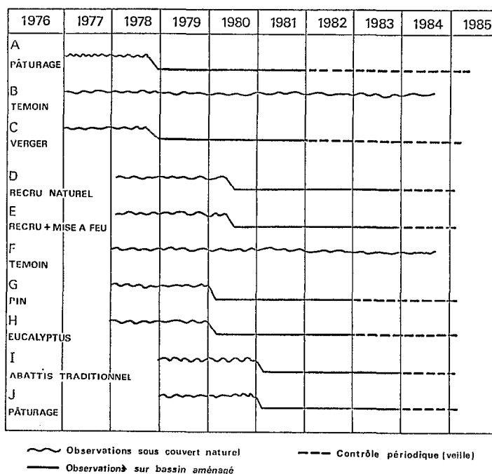
Fig. 2. — Ecérex Projet d'aménagement des bassins versants expérimentaux
