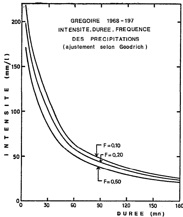
Fig. 5. — Fréquence des intensités des précipitations en fonction de leur durée à Grégoire, durant la période 1968-1976
