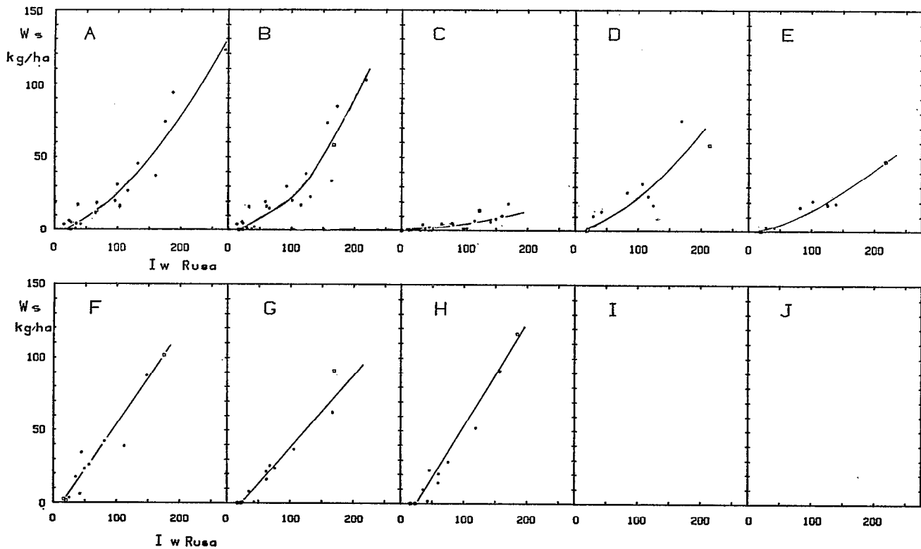
Fig. 8 A. — Ecérex 1977-1978, mensuel. Corrélations entre les quantités de matières en suspension (kg/ha) exportées mensuellement des bassins versants et la somme mensuelle des indices de Wischmeyer (RUSA) des précipitations. Les carrés... (idem fig. 1 A)
