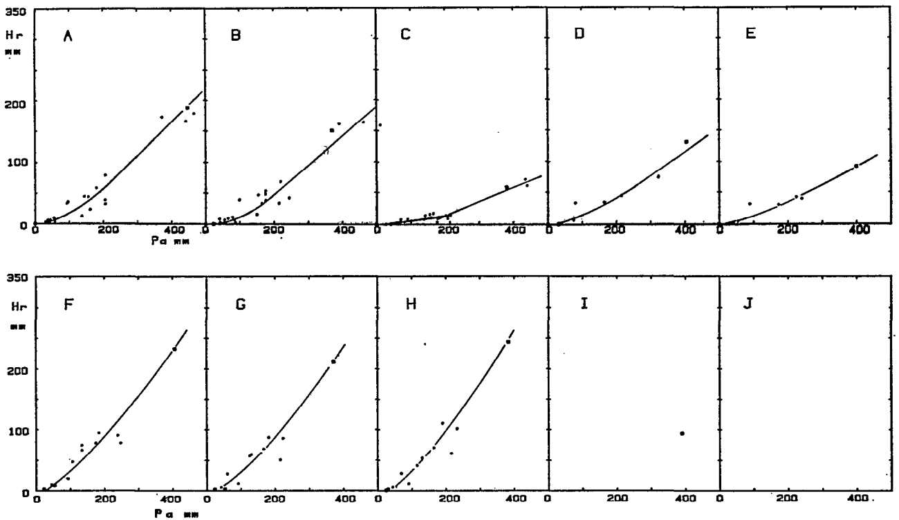
Fig. 2 A. — Ecérex 1977-1978, mensuel. Corrélations entre la lame ruisselée mensuelle (mm) et la hauteur mensuelle des averses ayant provoqué le ruissellement (mm) sur les bassins versants A à I. Les carrés clairs sont représentatifs... (idem fig. 1 A)
