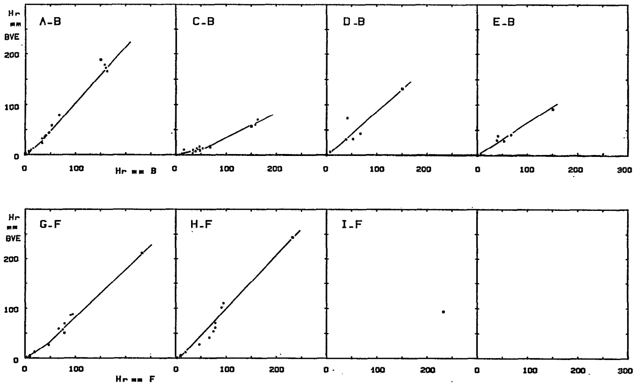
Fig. 4 A. — Ecérex 1977-1978, mensuel. Corrélations entre les lames ruisselées mensuelles (mm) sur les bassins versants expérimentaux et sur les bassins versants témoins B ou F. Les carrés clairs... (idem fig. 1 A)
