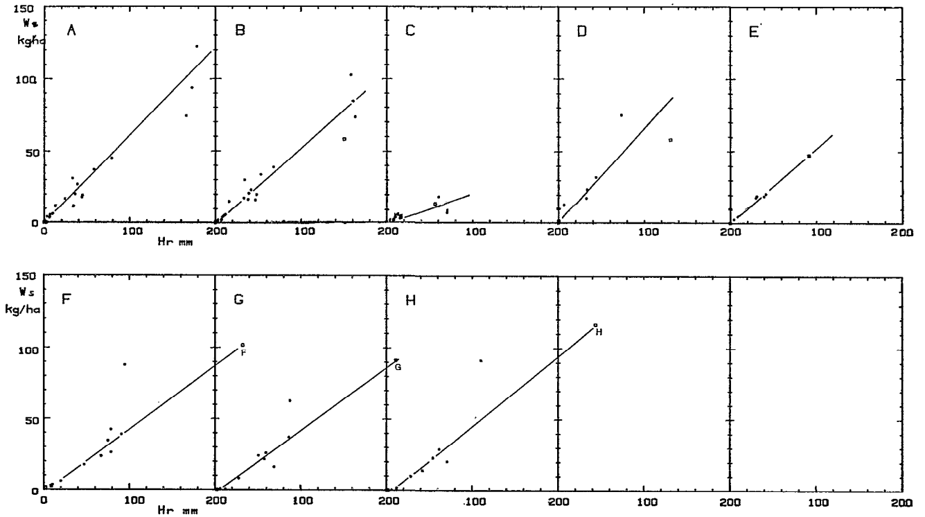
Fig. 9 A. — Ecérex 1977-1978, mensuel. Corrélations entre les quantités de matières en suspension (kg/ha) exportées mensuellement des bassins versants et la lame ruisselée mensuelle (mm). Les carrés clairs... (idem fig. 1 A)
