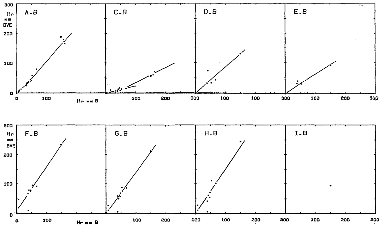
Fig. 5 A. — Ecérex 1977-1978, mensuel. Corrélations entre les lames ruisselées mensuelles (mm) sur les bassins versants et sur le bassin versant témoin B. Les carrés clairs... (idem fig. 1 A)
