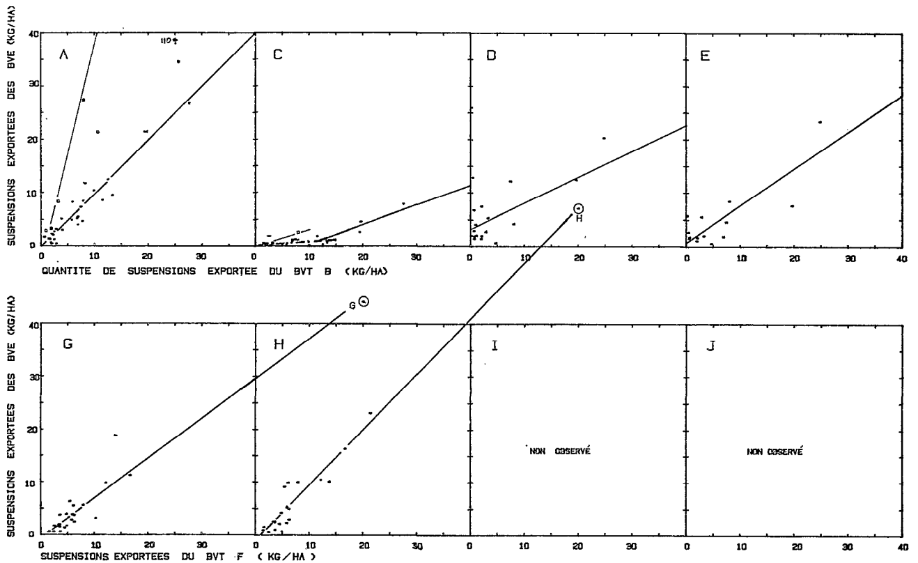
Fig. 10 A. — Ecérex 1977-1978, crues. Corrélations entre les quantités de matières en suspension (kg/ha) exportées au cours des crues sur les bassins versants expérimentaux et les bassins versants témoins B et F. Les carrés clairs... (idem fig. 1 A)
