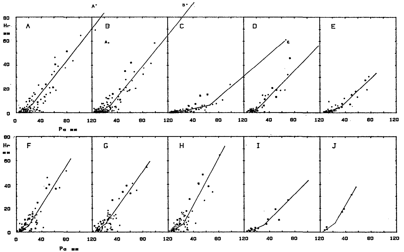
Fig. 1 A. — Ecérex 1977-1978, crues. Corrélations entre la lame ruisselée (mm) par crue et la hauteur de l'averse correspondante (mm), sur les bassins versants A à J. Les carrés clairs sont représentatifs d'événements intervenus à compter d'octobre 1978, date de la déforestation des bassins A et C. (Réduction 0,63 du graphique obtenu directement sur calculateur - traceur Hewlett-Packard de la série 98)
