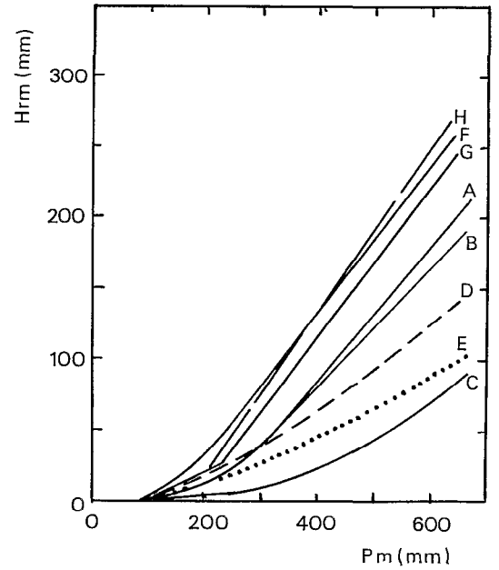
Fig. 9. — Ecérex 1977-1978. Corrélation entre la lame ruisselée mensuelle et la pluviométrie mensuelle sur les différents bassins
