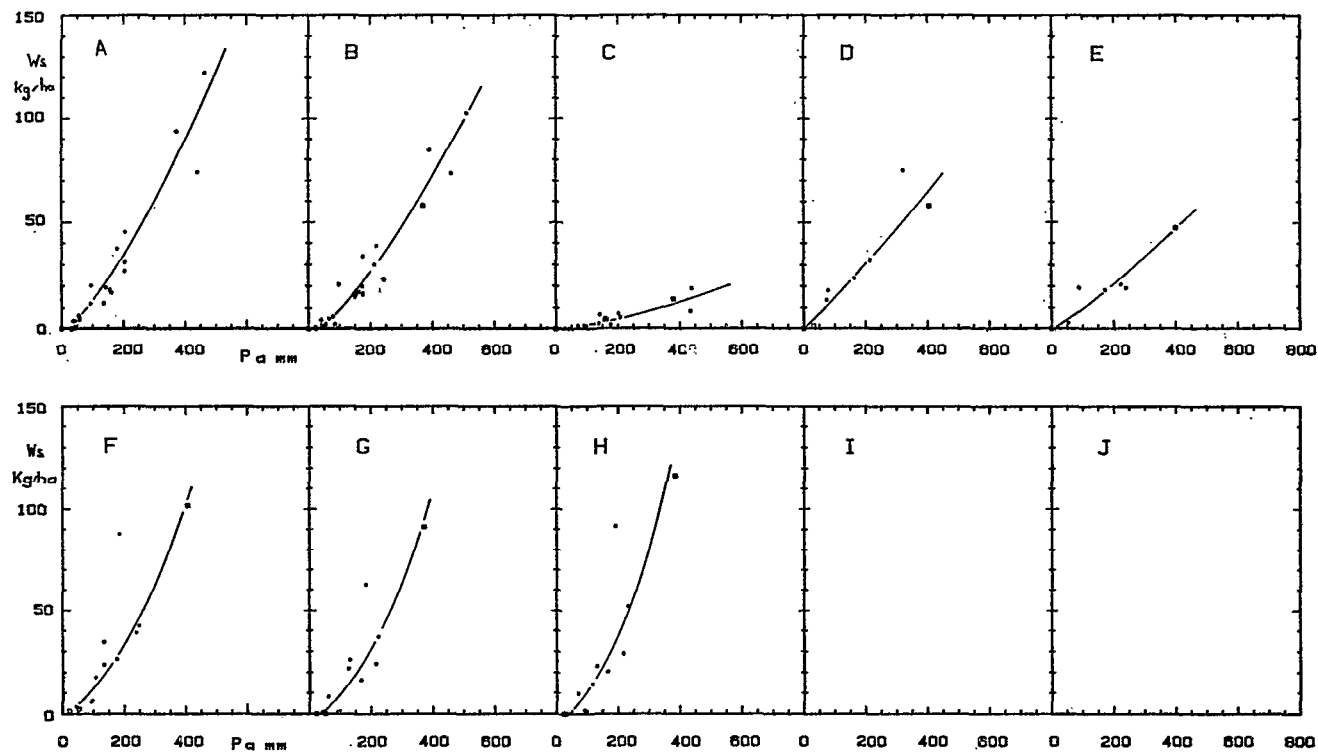
Fig. 6 A. — Ecérex 1977-1978, mensuel. Corrélations entre les quantités de matières en suspension (kg/ha) exportées mensuellement des bassins versants et la hauteur mensuelle des averse (mm) ayant provoqué le ruissellement. Les carrés... (idem fig. 1 A)
