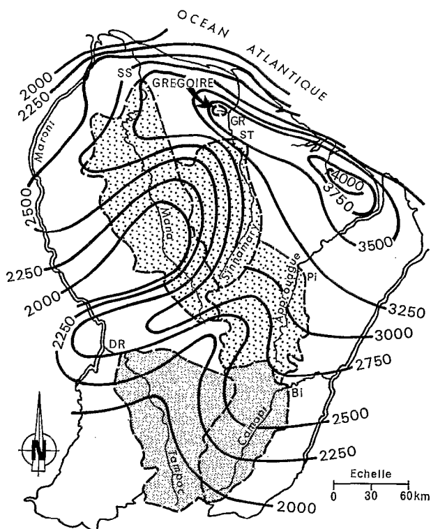
Fig. 1. — Pluviométrie moyenne annuelle (mm) en Guyane durant la période 1956-1976 (d'après Atlas de Guyane) Situation des bassins versants
