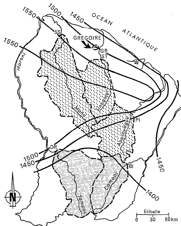
Fig. 2. — Evapotranspiration réelle moyenne annuelle (mm) en Guyane, estimée selon la méthode de Thornthwaite sur la période 1956-1960, d'après H. MADEC, 1963
