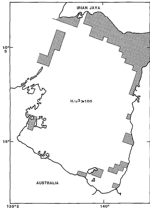
FIG. 6. — Areas of the Gulf of Carpentaria where the tidal mixing criterion ( H/u^3 ) is less than 100. These are shaded. Régions du Golfe dans lesquelles le critère de mélange dû à la marée ( H/u^3 ) est inférieur à 100. Ces régions sont ombrées
