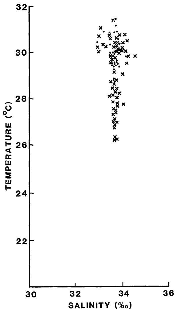
FIG. 4. — T.S. diagram for summer. See Figure 2 for details Diagramme T.S. d'été. Voir Figure 2 pour l'explication des symboles
