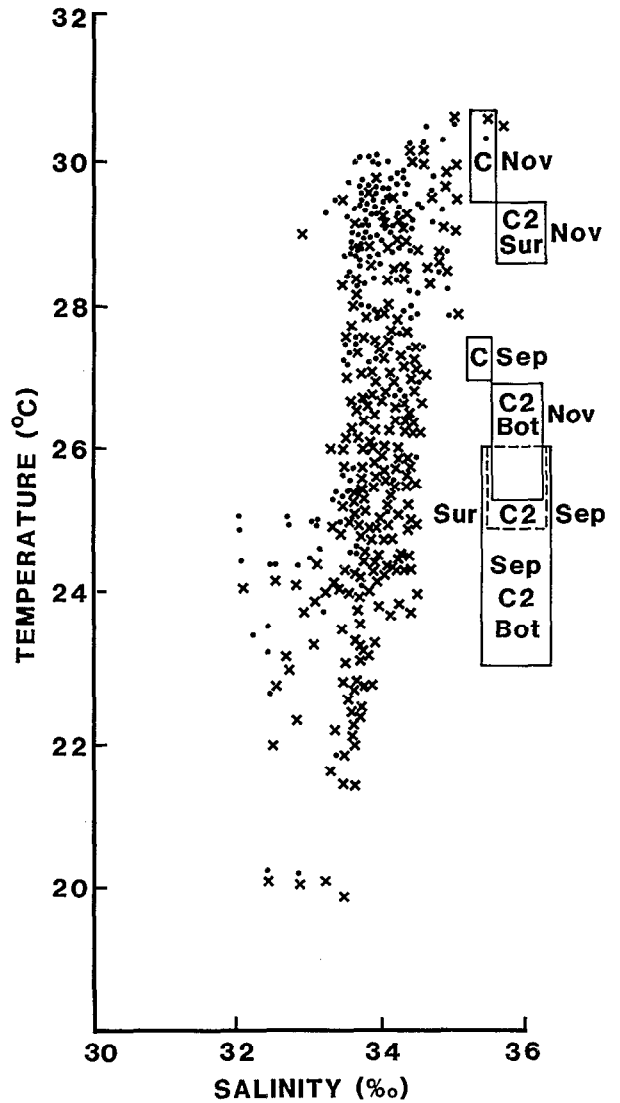
FIG. 3. — T.S. diagram for spring. See Figure 2 for details Diagramme T.S. de printemps. Voir Figure 2 pour l'explicitation des symboles
