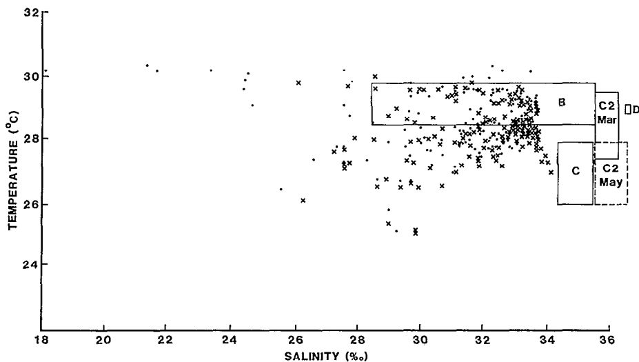
Fig. 5. — T.S. diagram for autumn. See Figure 2 for details Diagramme T.S. d'automne. Voir Figure 2 pour l'explicitation des symboles
