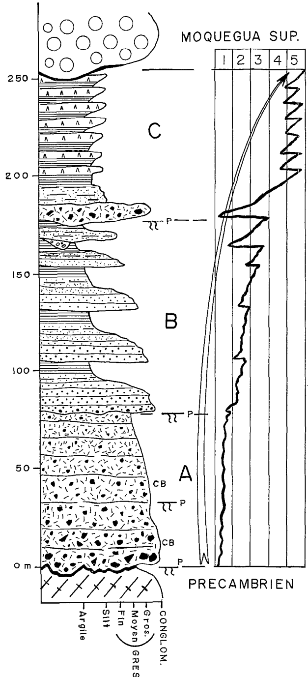
FIG. 7. — Formation Moquegua inférieure, coupe de la Mine La Eugenia. Mêmes symboles qu'en figure 6
