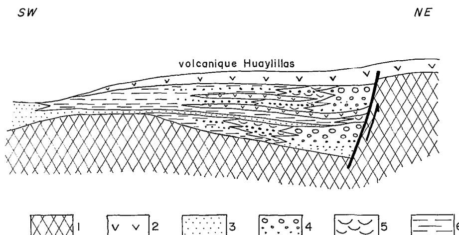
Fig. 15. — Modèle du bassin Moquegua supérieur, le long d'une transversale NE-SW, d'après MAROCCO et al. , 1984, modifié. 1 : substratum ; 2 : volcanisme ; 3 : marin ; 4 : cônes ; 5 : fluvatile ; 6 : lacustre et palustre
