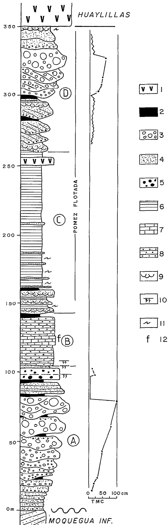
FIG. 12. — Formation Moquegua supérieur, coupe de Cuno-Cuno, d'après MAROCCO et al. , 1984. Pomez flotada : ponce flottée. TMC : diamètre du plus gros grain. 1 : volcanisme explosif; 2 : argiles; 3 : conglomérats; 4 : grès fluviale; 5 : coulée de boue; 6 : dépôts lacustres; 7 : calcaires marins; 8 : grès littoraux; 9 : stratification croisée; 10 : pédogenèse; 11 : slumps; 12 : fossiles
