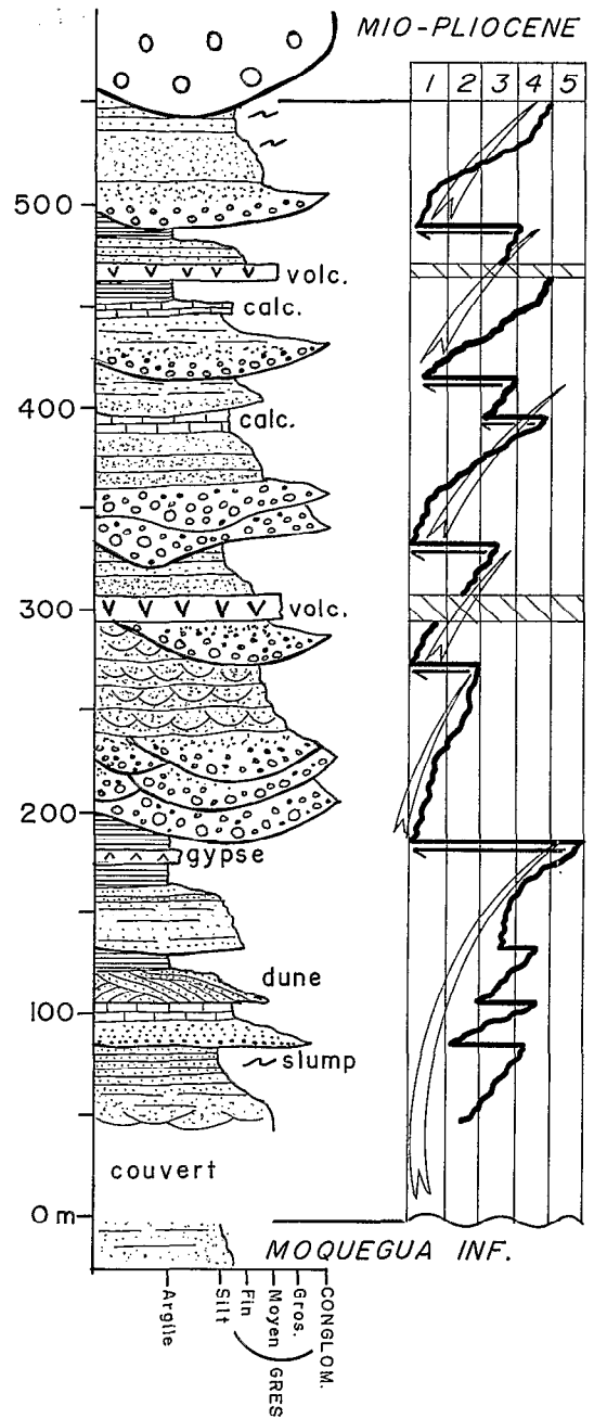
FIG. 13. — Formation Moquegua supérieur, coupe du rio Majes. 1 : Cônes alluviaux; 2 : Fluviale; 3 : palustre; 4 : lacustre; 5 : évaporites
