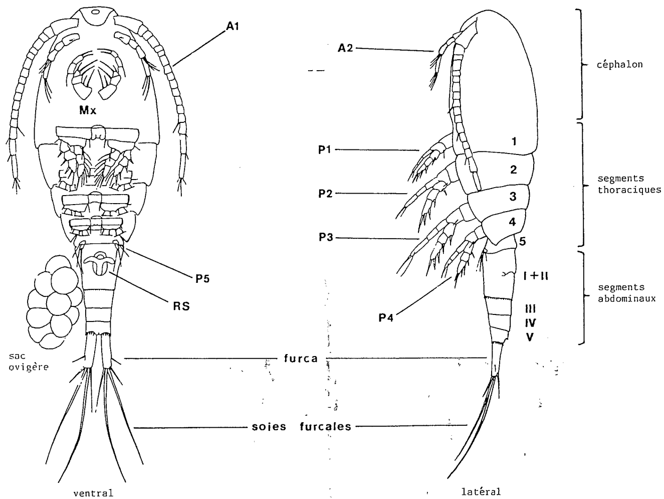
Fig. 3: Morphologie d'un cycloptide (femelle de Thermocyclops inopinus ).
