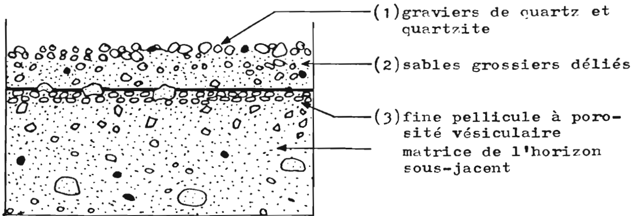
Type 21 SURFACE A RECOUVREMENT DE SABLES GROSSIERS
