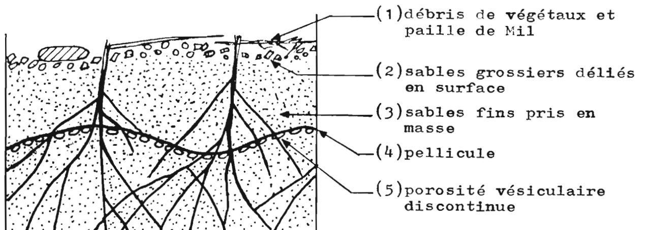
Type 37 SURFACE A RECOUVREMENT SABLEUX EOLIEN ENHERBEE SUR DUNES ET AVAL DE JUPES DE PIEMONT
