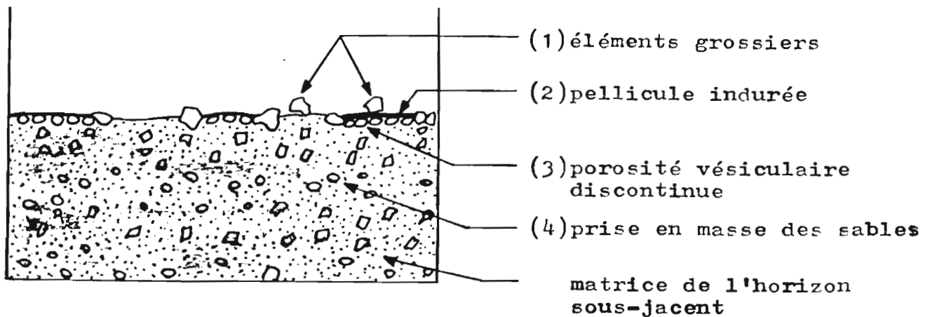
Type 41 SURFACE A PELLICULE PLASMIQUE ET ELEMENTS GROSSIERS ENCHASSES
