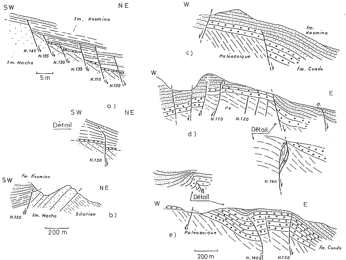
Fig. 4. — Exemples de déformations synsédimentaires. Exemples of synsedimentary deformations
