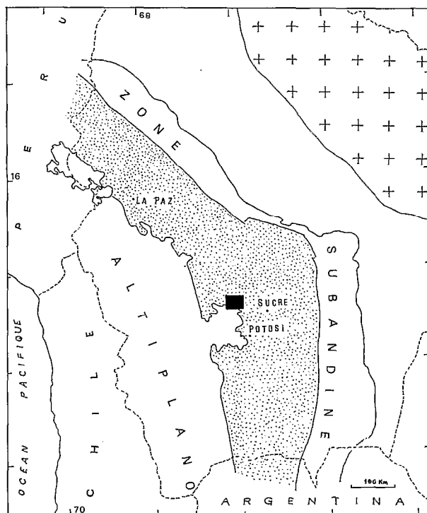
Fig. 1. — Situation du secteur étudié dans la Cordillère Orientale de Bolivie. Sketch map of the study area in the Eastern Cordillera of Bolivia
