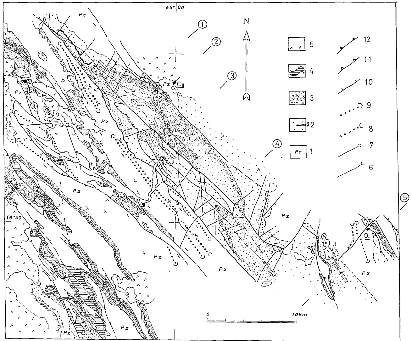
Fig. 2a. — Carte géologique de la région de Macha. Geological map of the region of Macha
