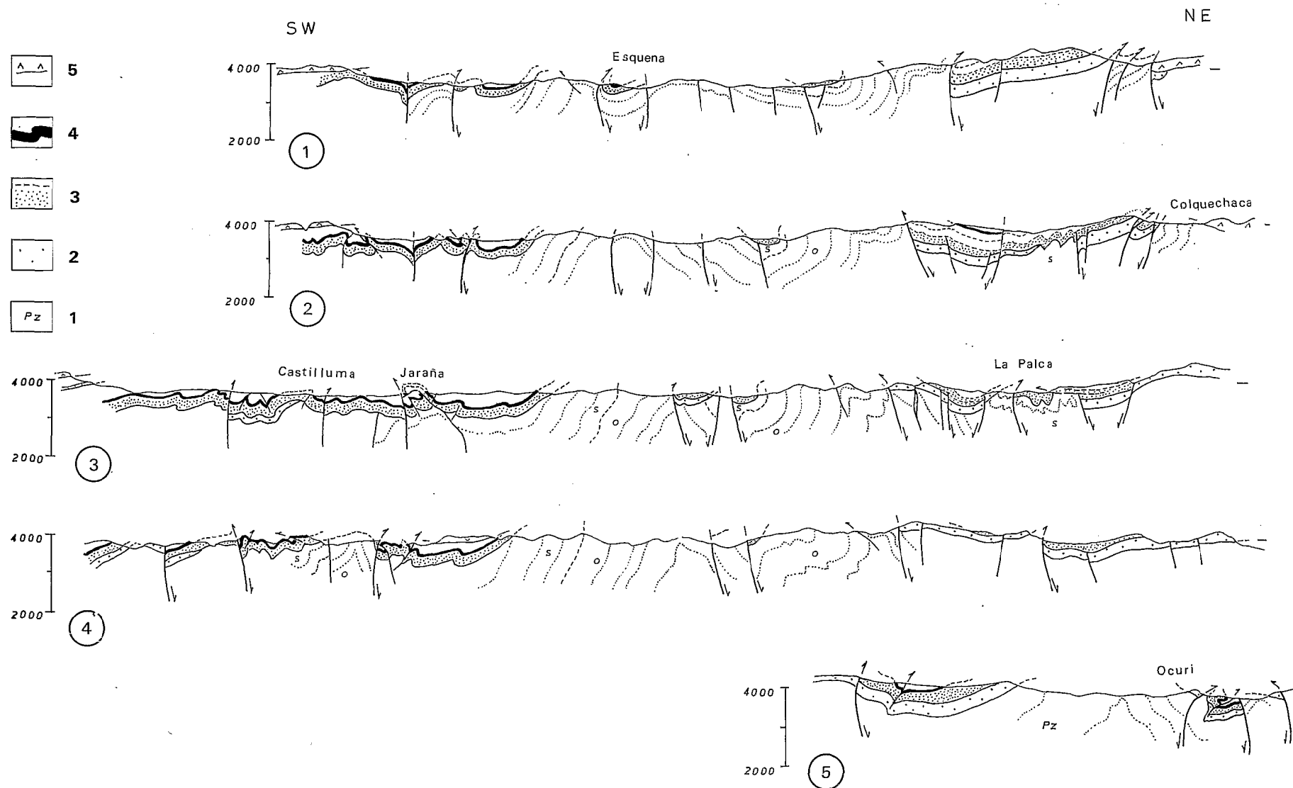
Fig. 2b. — Coupes de la région de Macha, (cf. légende fig. 2a). Sections of the region of Macha
