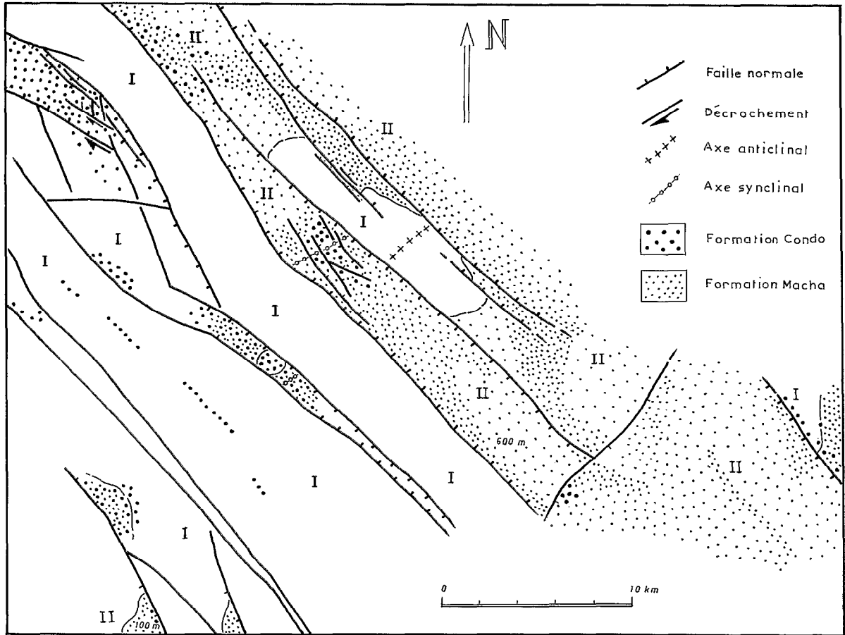
Fig. 3. — Écorché géologique antérieur au dépôt de la formation Kosmina discordante sur le Paléozoïque (I) ou sur la formation Macha (II). Les conglomérats Condo sont représentés qui, par endroit, marquent la base de la formation Kosmina. Geological sketch map before deposit of the unconformable formation on (I) paleozoic terrace, on (II) on formation Macha. The Condo conglomerates are also shown if existent and figure the base of the Kosmina formation
