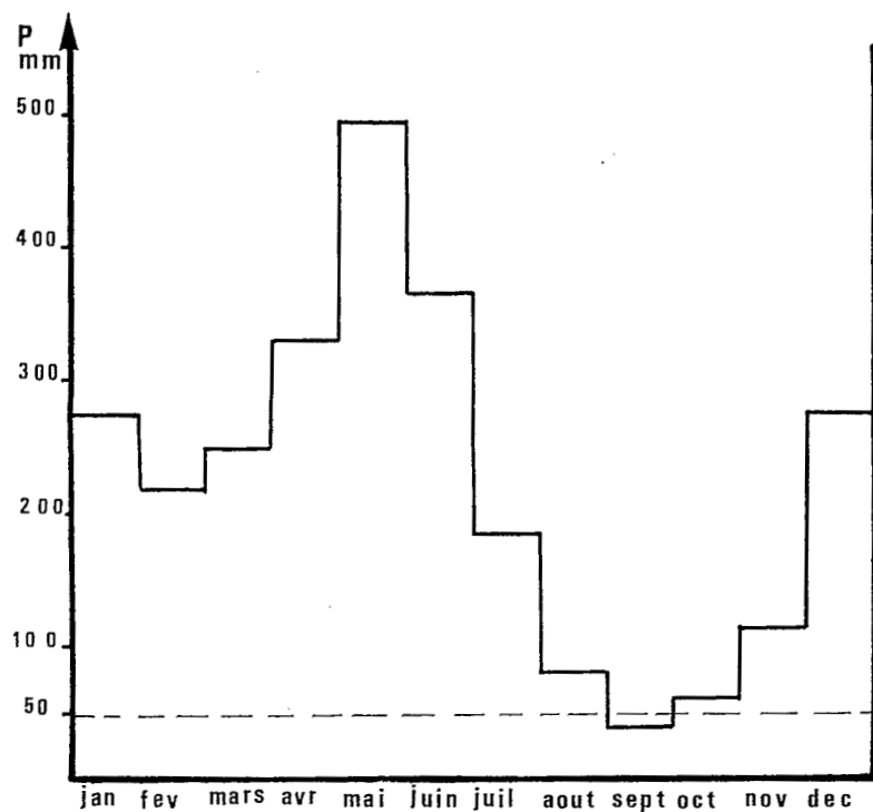
Fig. 1: Pluviométrie moyenne mensuelle à Sinnamary sur la période 1953-1987 (le mois de septembre qui reçoit moins de 50 mm est considéré comme sec).
