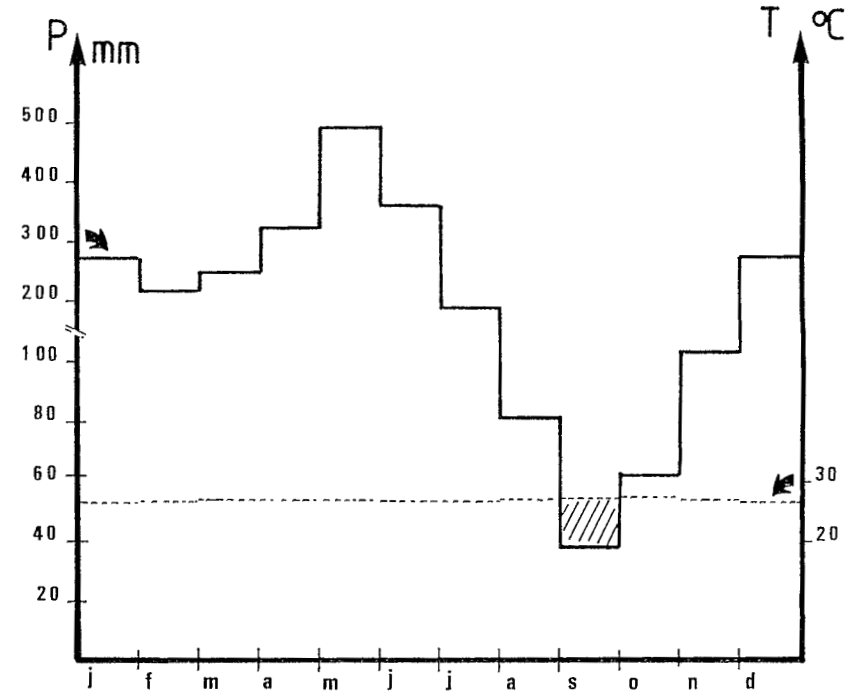
Fig. 2: Diagramme ombrothermique pour l'année climatique moyenne à Sinnamary (le mois de septembre où le graphe des pluies passe sous le graphe des températures est considéré comme sec). Voir le texte pour les conventions d'échelle.
