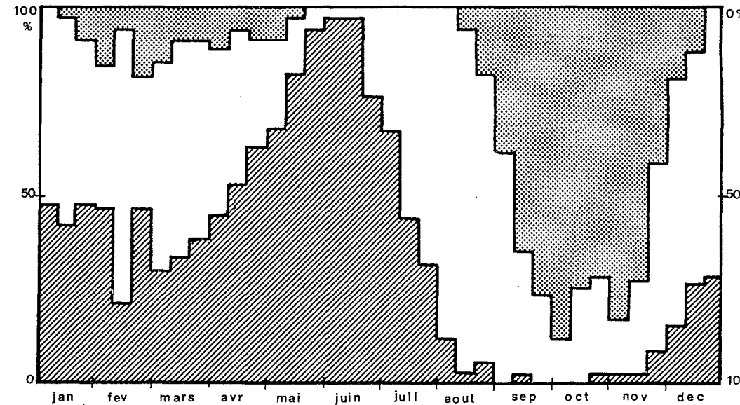
Fig. 3: Fréquence des périodes sèches (en pointillé, en haut), hyperhumides (en hachures, en bas) et favorables (en clair, au milieu). Par exemple, la première décade de mars est statistiquement, sur 100 années, sèche 15 fois, trop humide 30 fois et favorable 55 autres fois.
