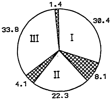
Figure 5. — Taux de similitude de peuplement (pourcentage de « recouvrement ») des espèces d'arbres de trois îlots forestiers du Parc National de la Comoé.
