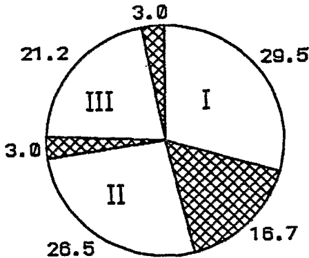
Figure 6. — Taux de similitude de peuplement (pourcentage de « recouvrement ») des espèces d'Oiseaux de trois îlots forestiers du Parc National de la Comoé.
