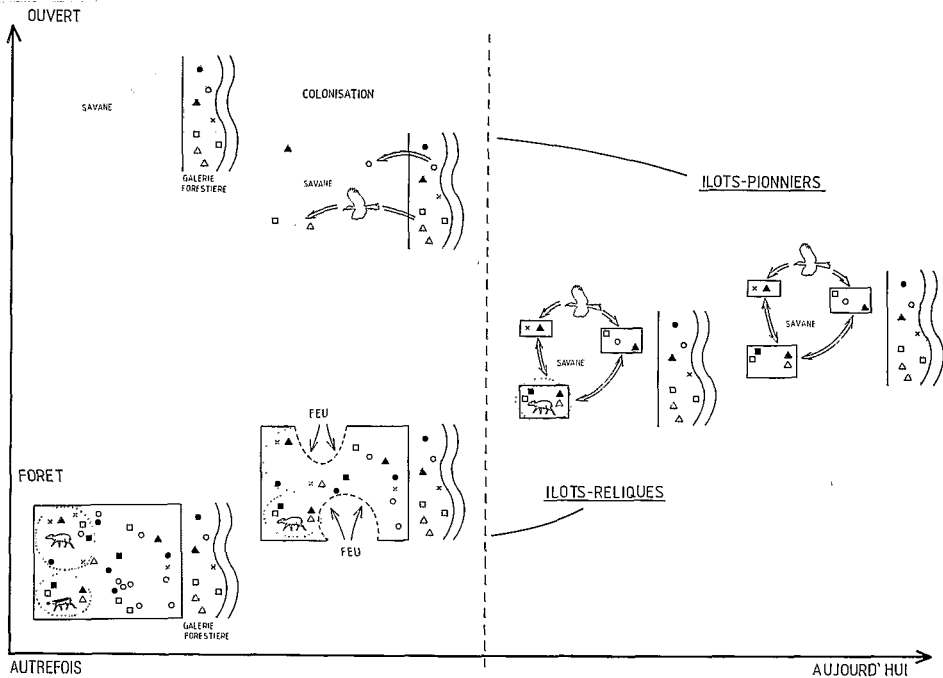
Figure 7. — Origine des îlots forestiers selon les deux hypothèses possibles sur leur origine : îlots-reliques ou îlots-pionniers. (D'après MÜHLENBERG, 1988a)
