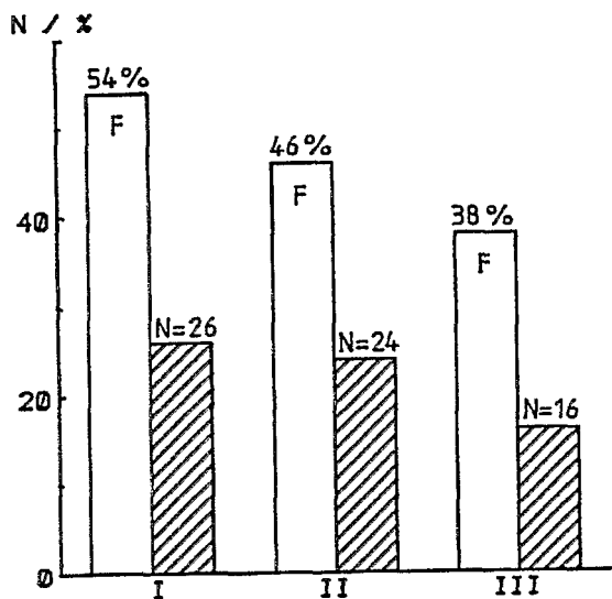
Figure 4. — Appartenance des espèces d'arbres et d'Oiseaux des trois îlots forestiers étudiés au Parc National de la Comoé. F : espèce de forêt humide (N = 41). En hachures : les espèces de savane.
