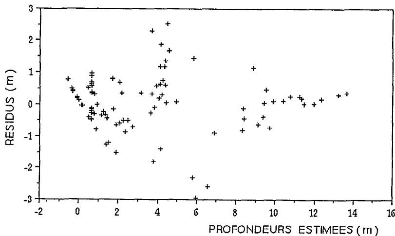
Fig. 11. — Représentation des profondeurs estimées par l'analyse en fonction des erreurs sur les mesures. Residual versus estimated water depth diagram.
