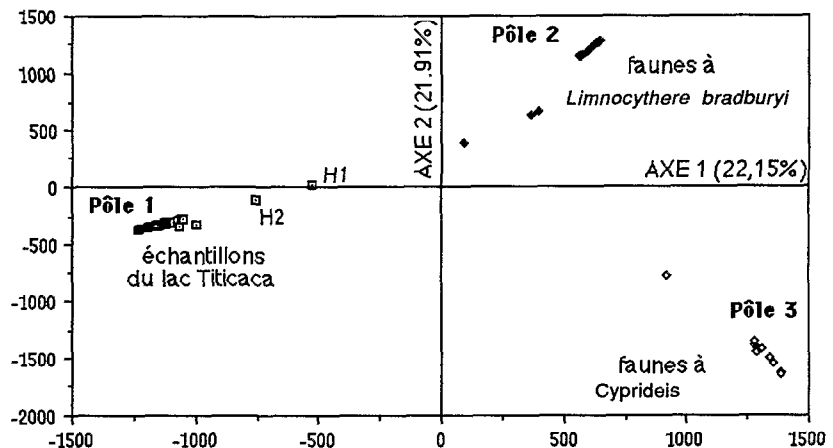
Fig. 2. — Projection des échantillons actuels sur le plan des 2 premiers facteurs de l'analyse.
