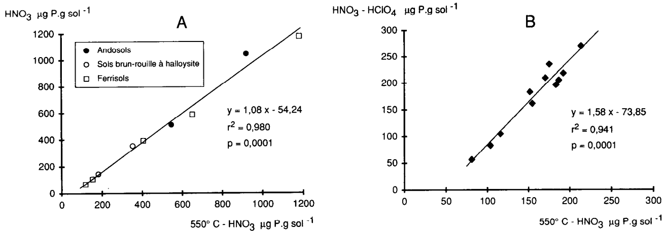
Fig. 1. – Relations entre la détermination du phosphore par la méthode calcination-acide nitrique et les méthodes acide nitrique (A : ferrisols, sols bruns à halloysite, andosols) et nitro-perchlorique (B : sols ferrugineux et ferrallitiques). Calcination-nitric acid method relations with nitric (A : ferrisols, halloysite brown soils, andosols) and nitro-perchloric method (B : ferrugineous and ferrallitics soils).
