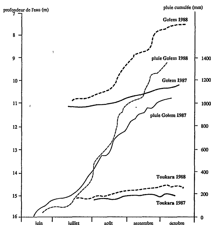
Fig. 7. - Comparaison des recharges 1987 et 1988 sur les puits de Golem et de Toukara (pluies cumulées et niveaux piézométriques) (Comparison of the 1987 and 1988 recharges on Golem and Toukara wells. (Cumulative rainfalls and piezometrical water levels))
